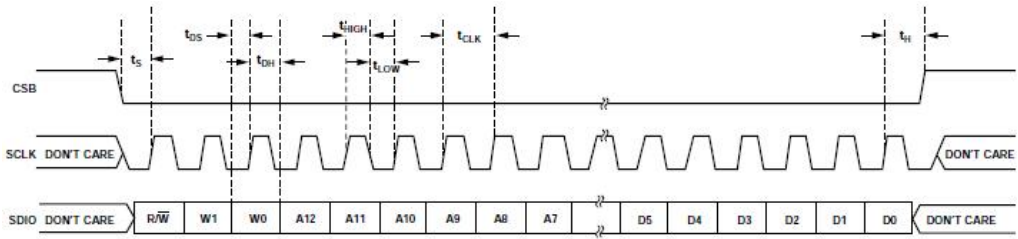
图 9.SPI 串行端口接口时序
