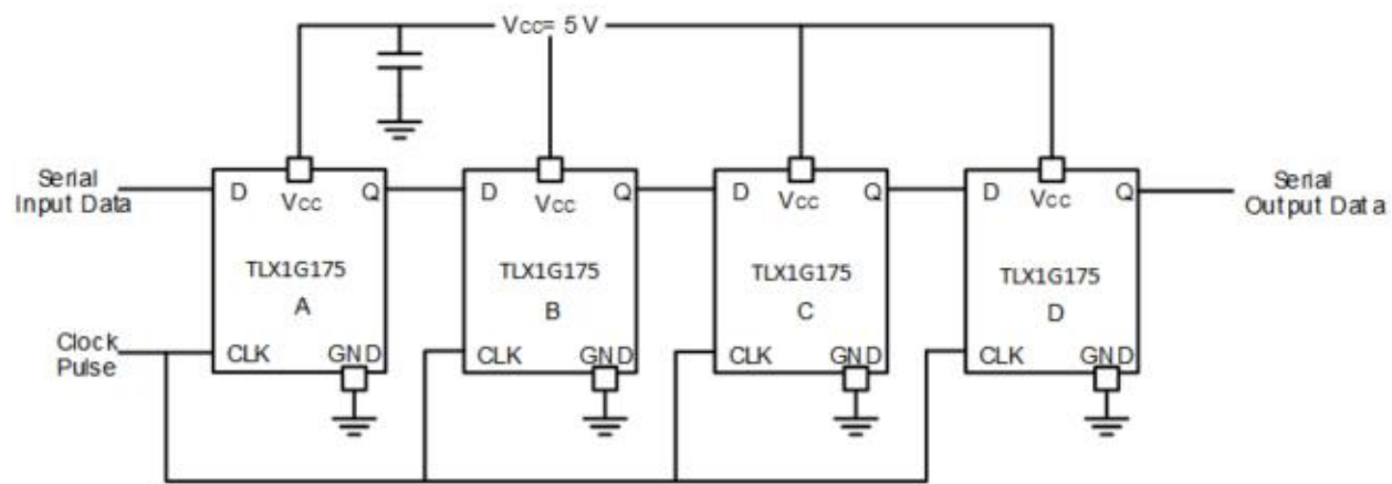
图 3.4 位串行移位寄存器
