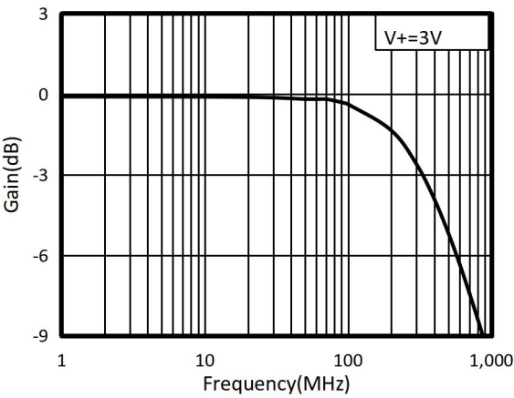
图 1. 带宽与频率
