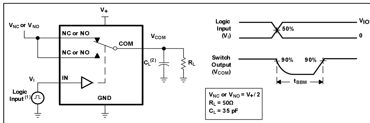
图 9. 先断后通时间 ( t_{BBM} )
