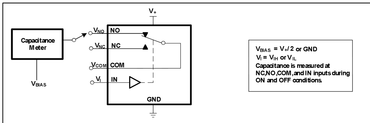
图 5.电容 ( C_I 、 C_{COM(ON)} 、 C_{NC(OFF)} 、 C_{NC(ON)} 、 C_{NO(OFF)} 、 C_{NO(ON)} )
