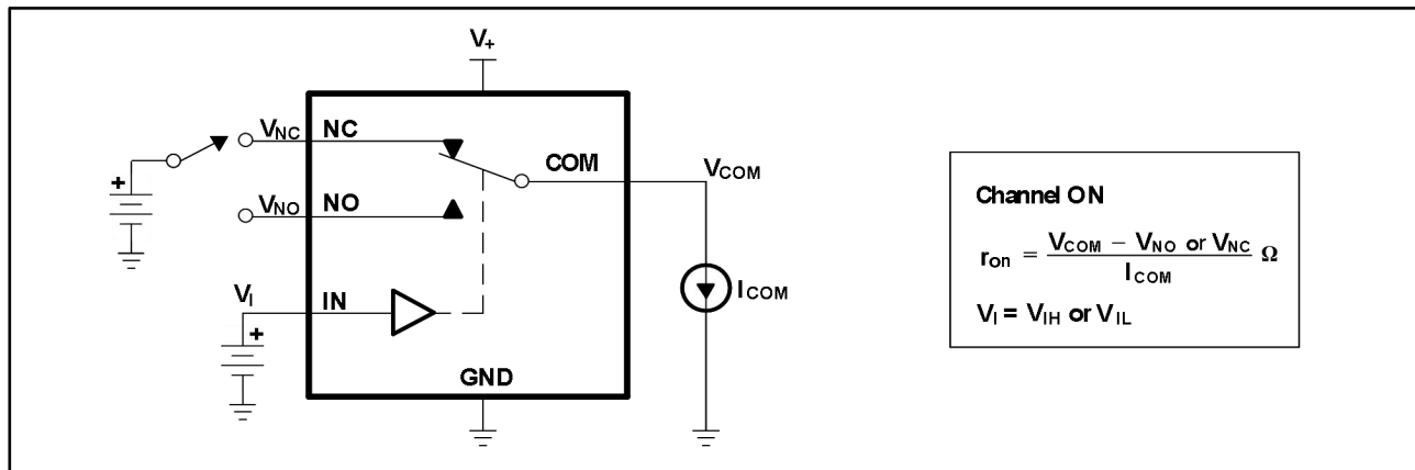
图 2. 导通电阻 ( R_{on} )
