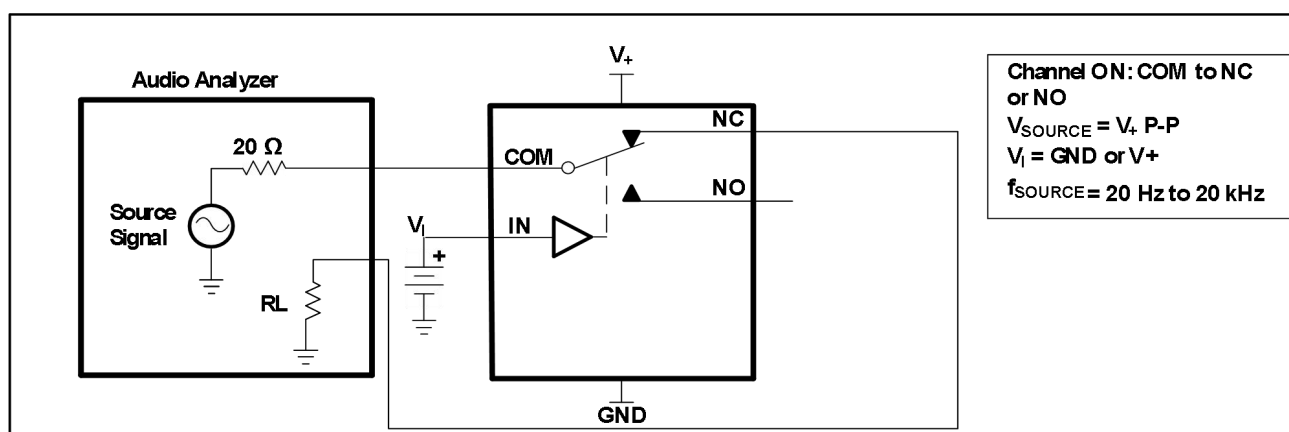
图 12. 总谐波失真 (THD)
