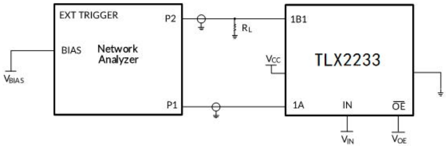
测试电路 3. 频率响应 (BW) 测试电路
