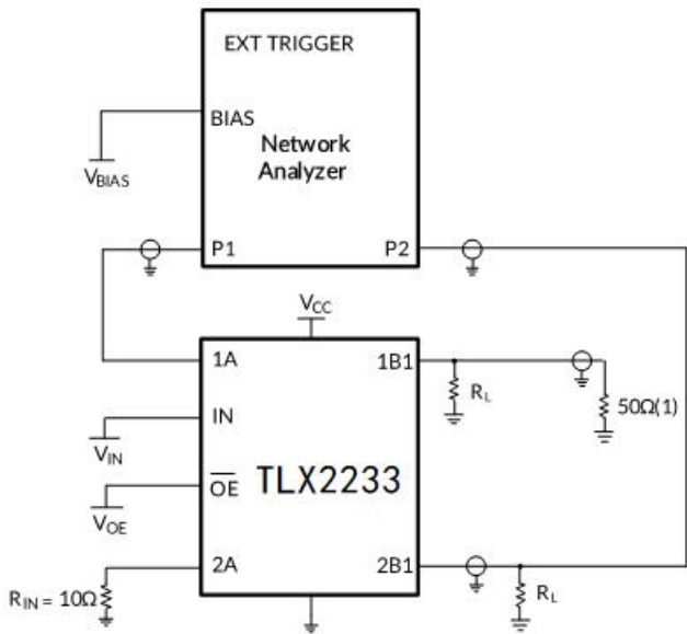
测试电路 3. 频率响应 (BW) 测试电路
