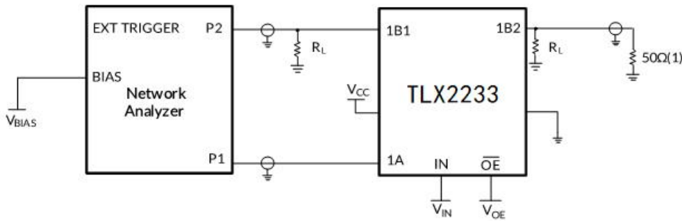
测试电路 5. 关断隔离测试电路 (OIRR)
