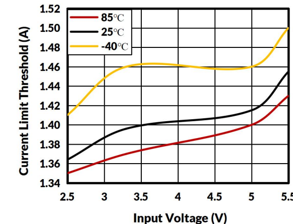
图 8. 电流限制阈值与输入电压的关系
