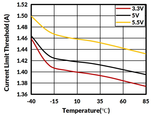
图 9. 电流限制阈值与温度的关系
