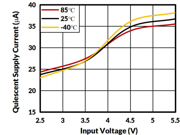
图 4. 静态电流与输入电压的关系
