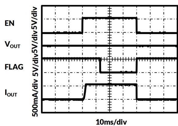
图 22. 器件启用短路
