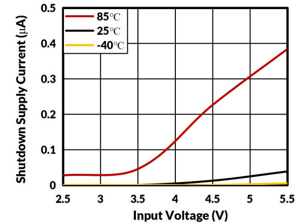
图 5. 关断电流与输入电压的关系
