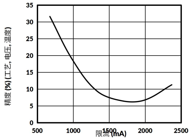
图 14. 电流限制精度与限流的关系
