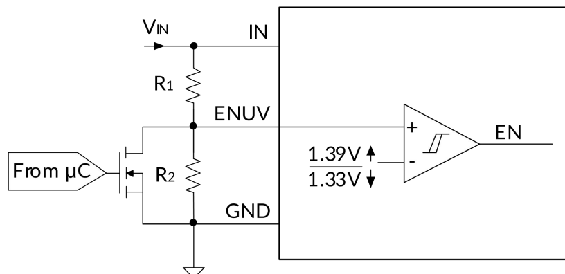
图 27. 关断控制
