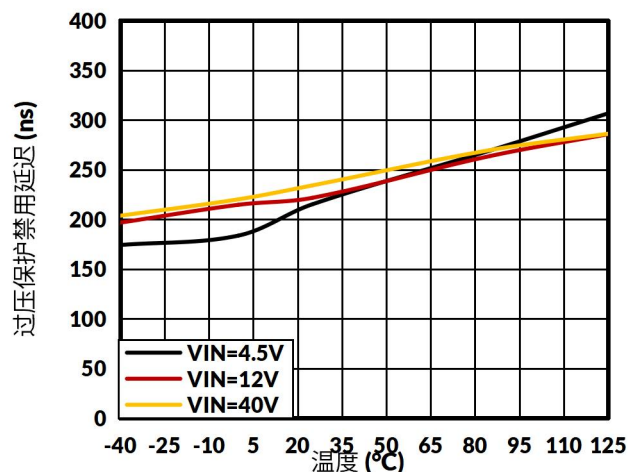
图 5. 过压保护禁用延迟 t_{ovp\_DLY} 与温度的关系
