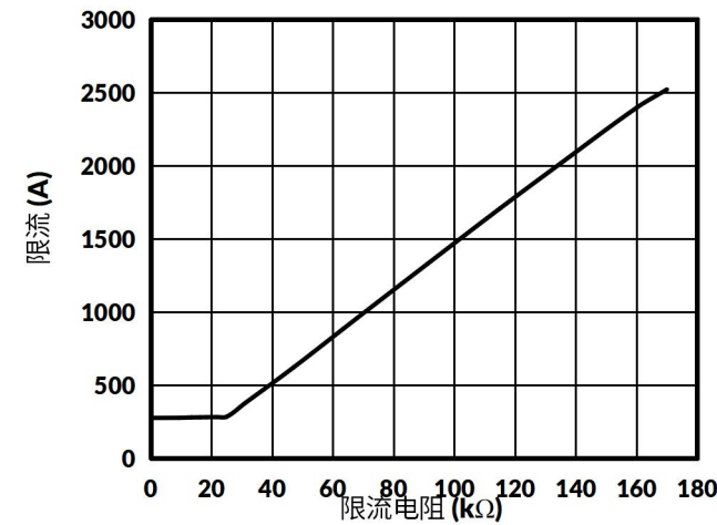
图 13. 限流与限流电阻的关系
