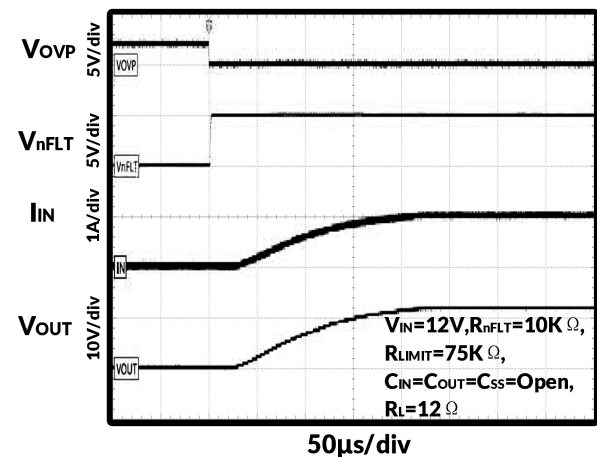
图 17. OVP 启动延迟: OVP ↓ 至输出斜坡 ↑
