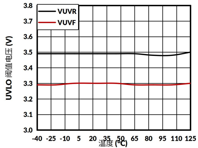
图 8. UVLO 阈值电压与温度的关系
