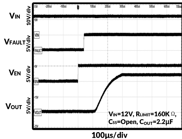
图 15. 使能启动
