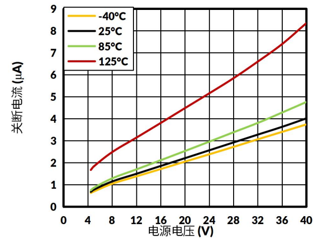
图 7. 关断电流与电源电压的关系
