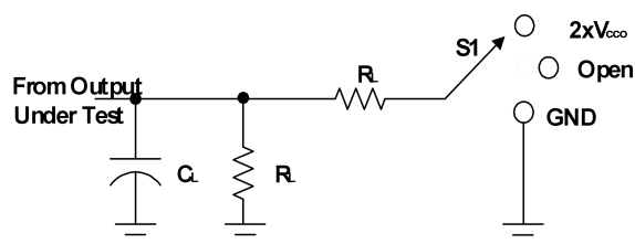
负载电路
