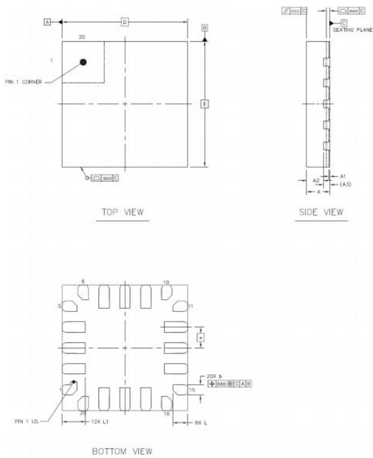
图 18 QFN20 封装图
