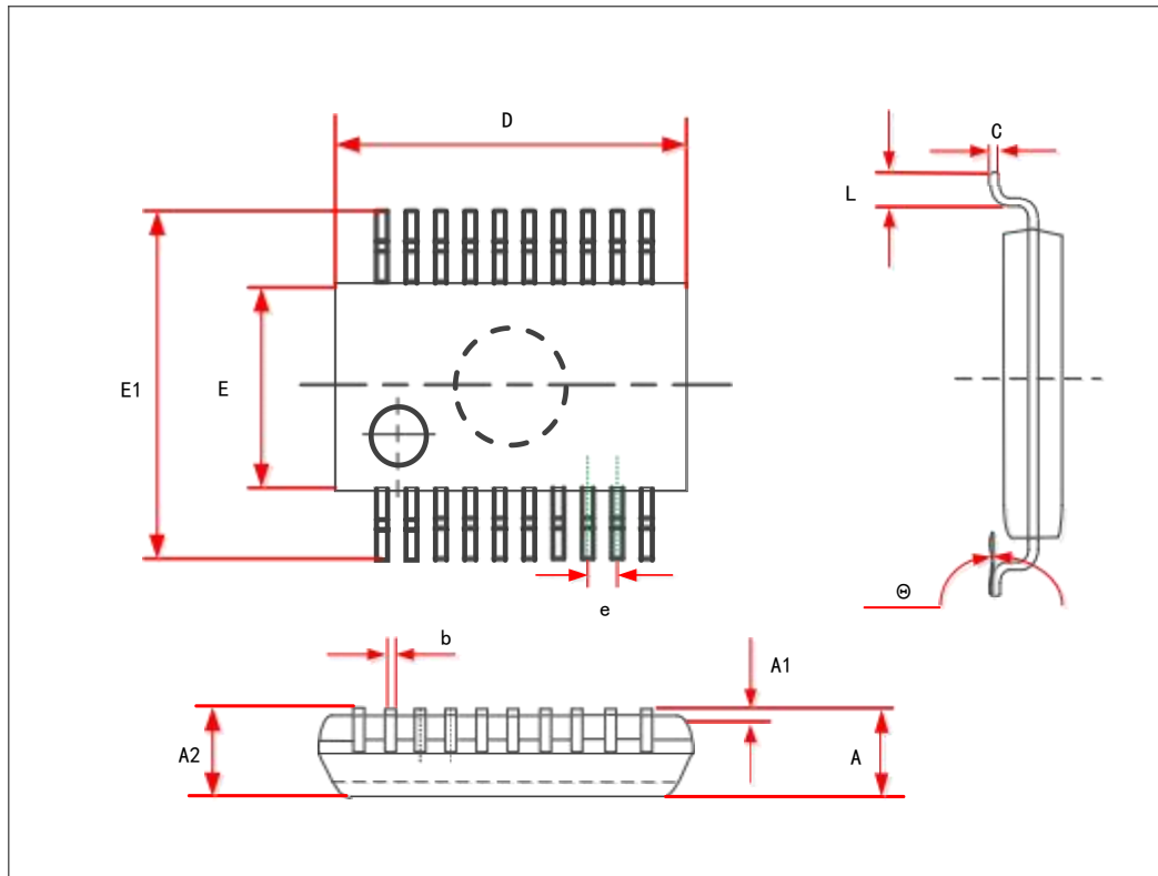
图 17 SOP20 封装图
