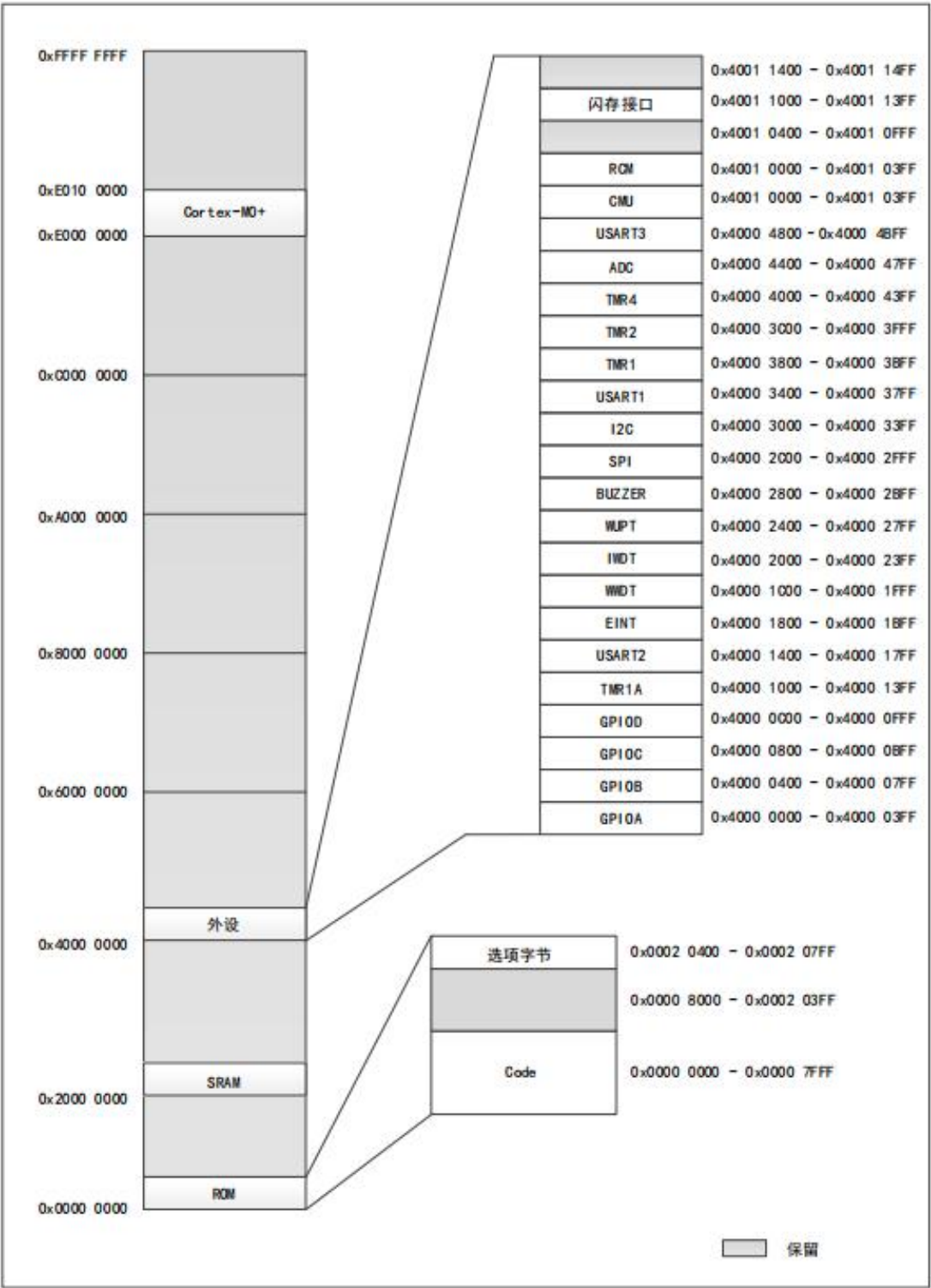
图 4 TLX32F003x4x6 系列地址映射图
