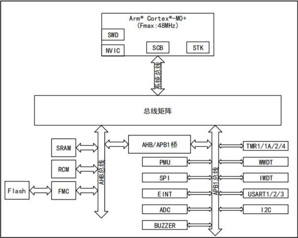
图 3 TLX32F003x4x6 系列系统框图
