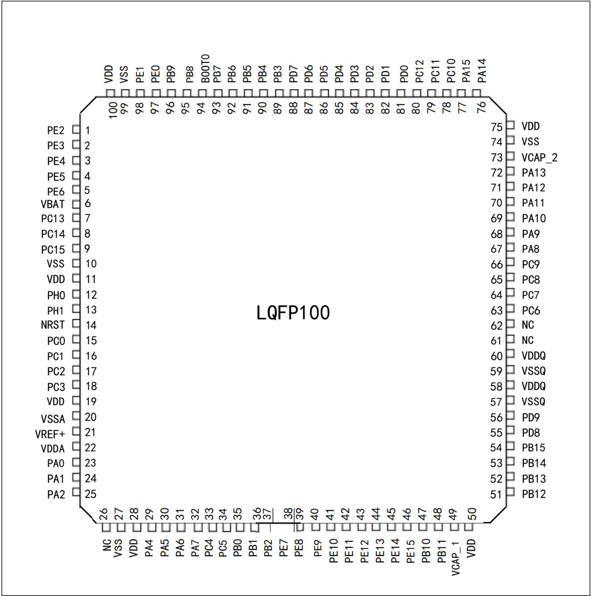
图 1 TLX32F407VGT6S 系列 LQFP100 引脚分布图
