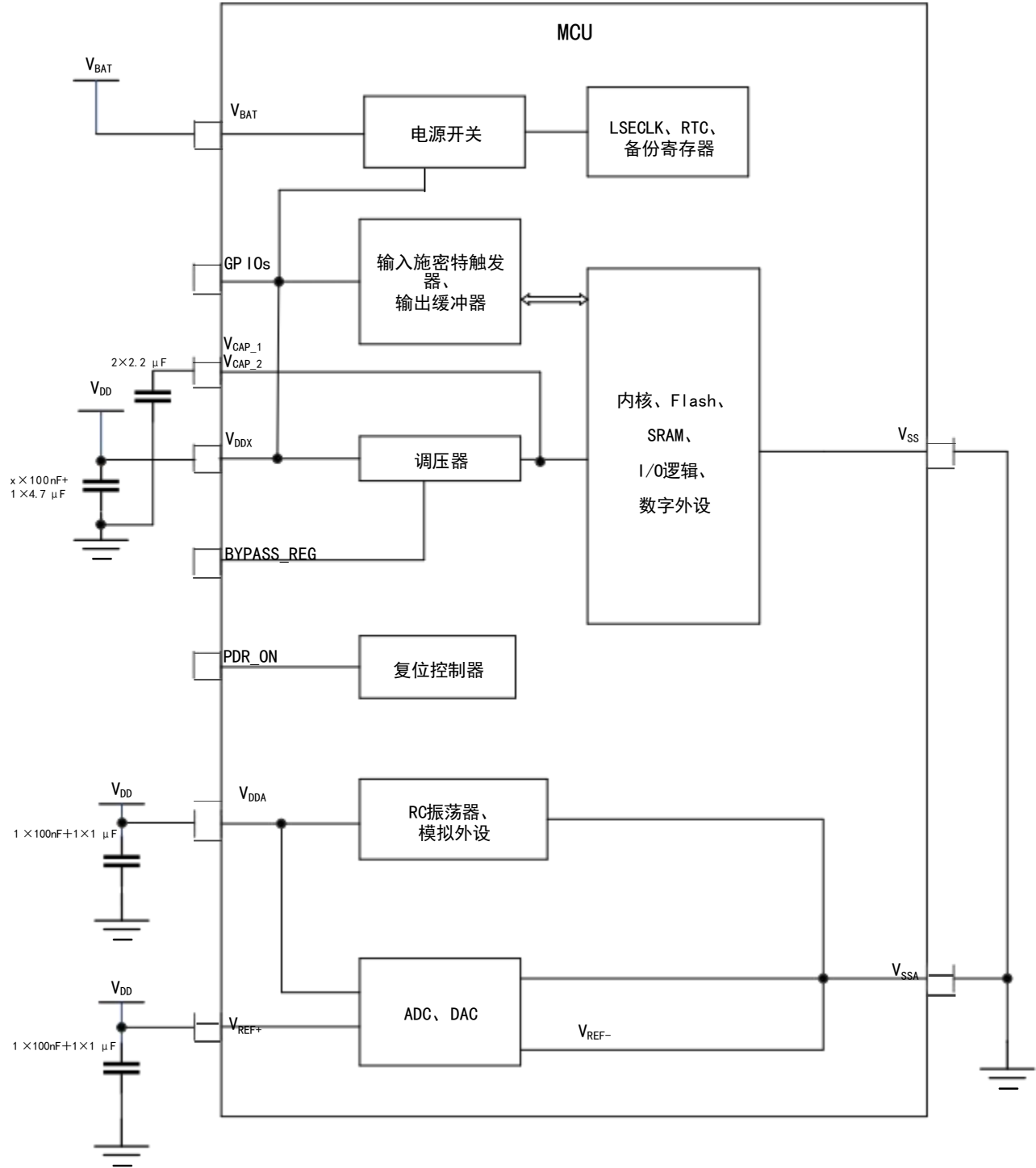
图 5 电源方案
