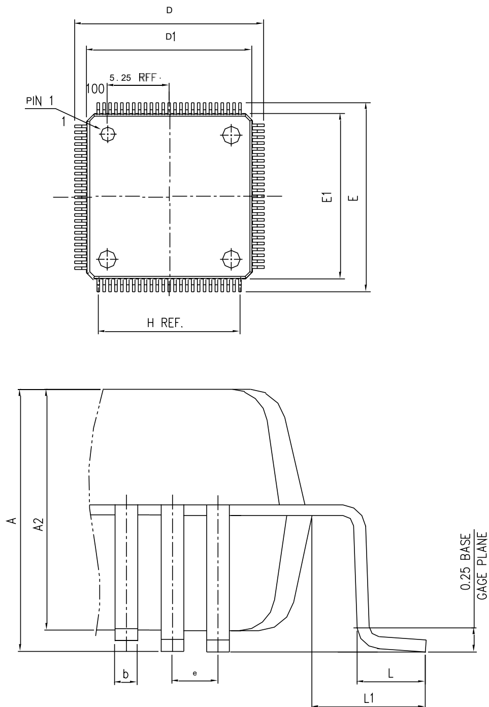
图 14 LQFP100 封装图
