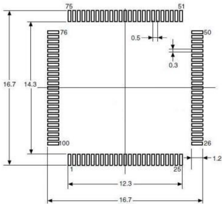
图 15 LQFP100 – 100 引脚，14 x 14mm 焊接 Layout 建议
