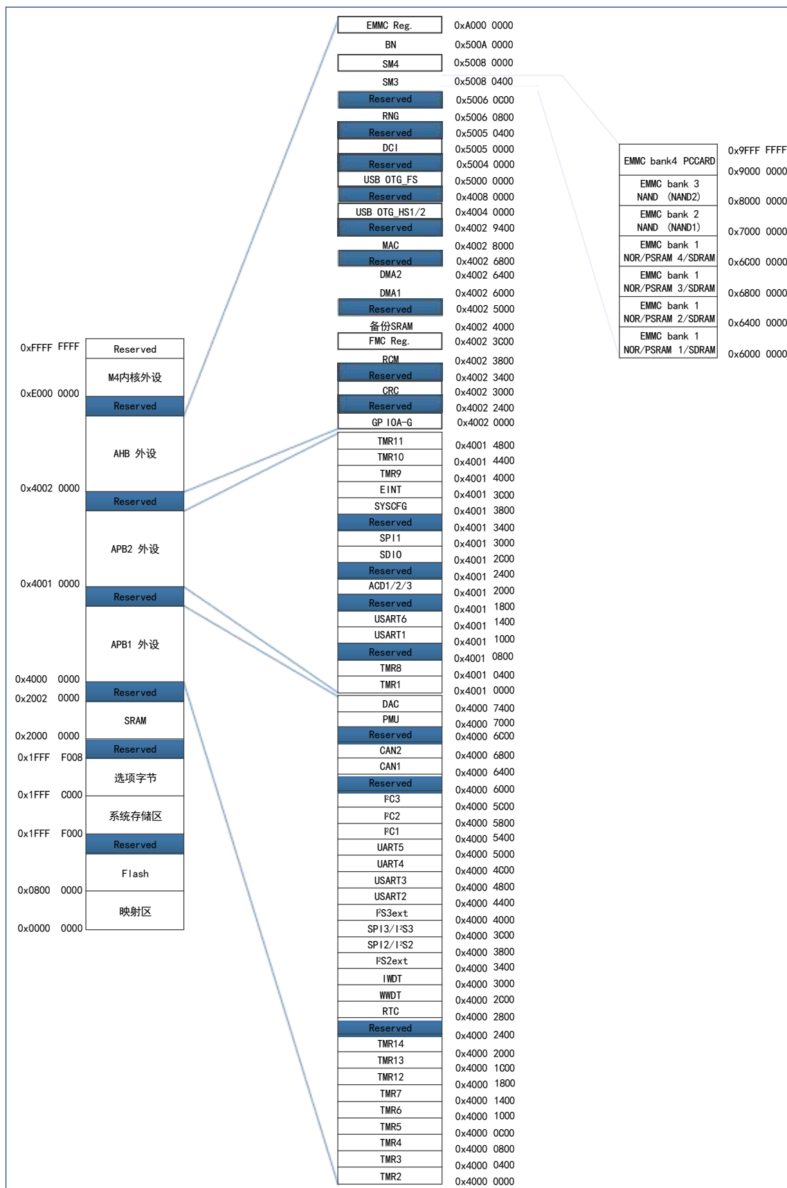
图 3 TLX32F407VGT6S 系列地址映射图
