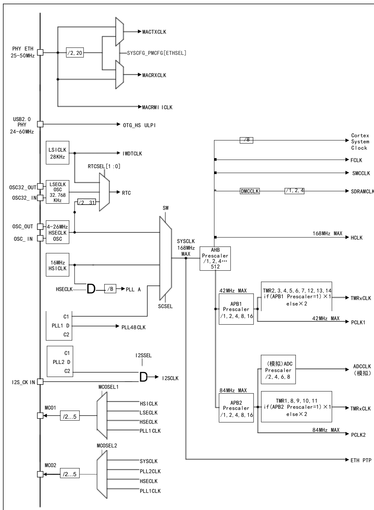
图 4 TLX32F407VGT6S 时钟树
