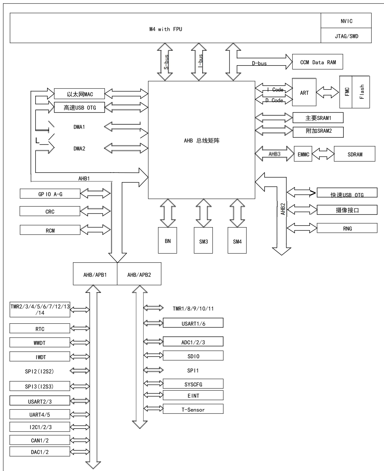
图 2 TLX32F407VGT6S 系统框图
