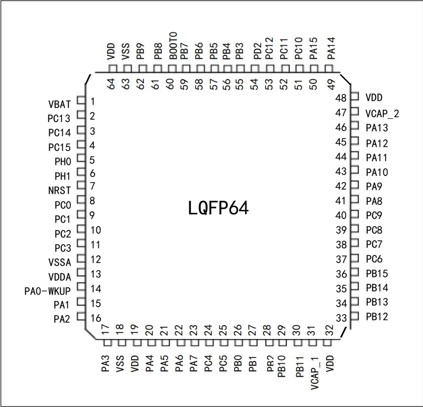
图 4 TLX32F407xG 系列 LQFP64 引脚分布图
