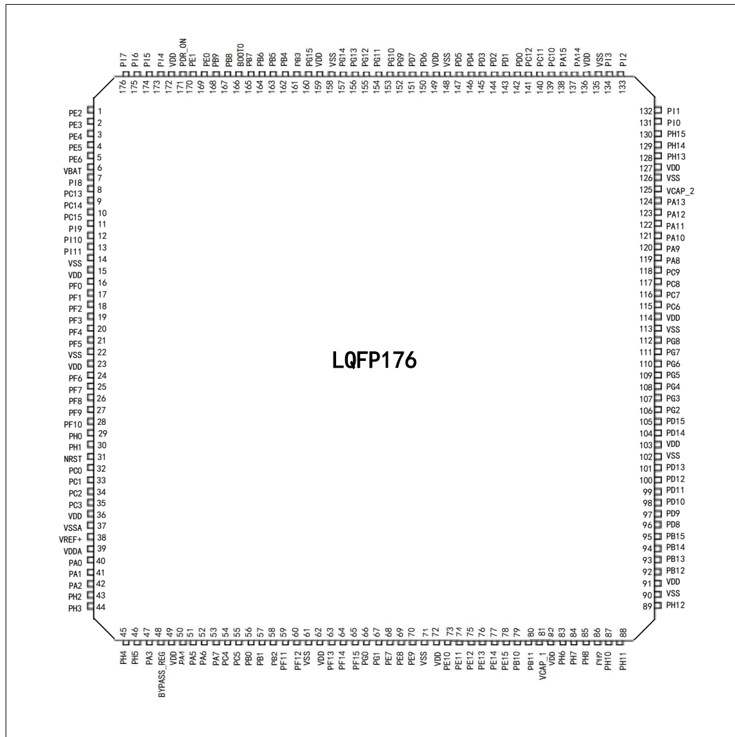
图 1 TLX32F407xG 系列 LQFP176 引脚分布图
