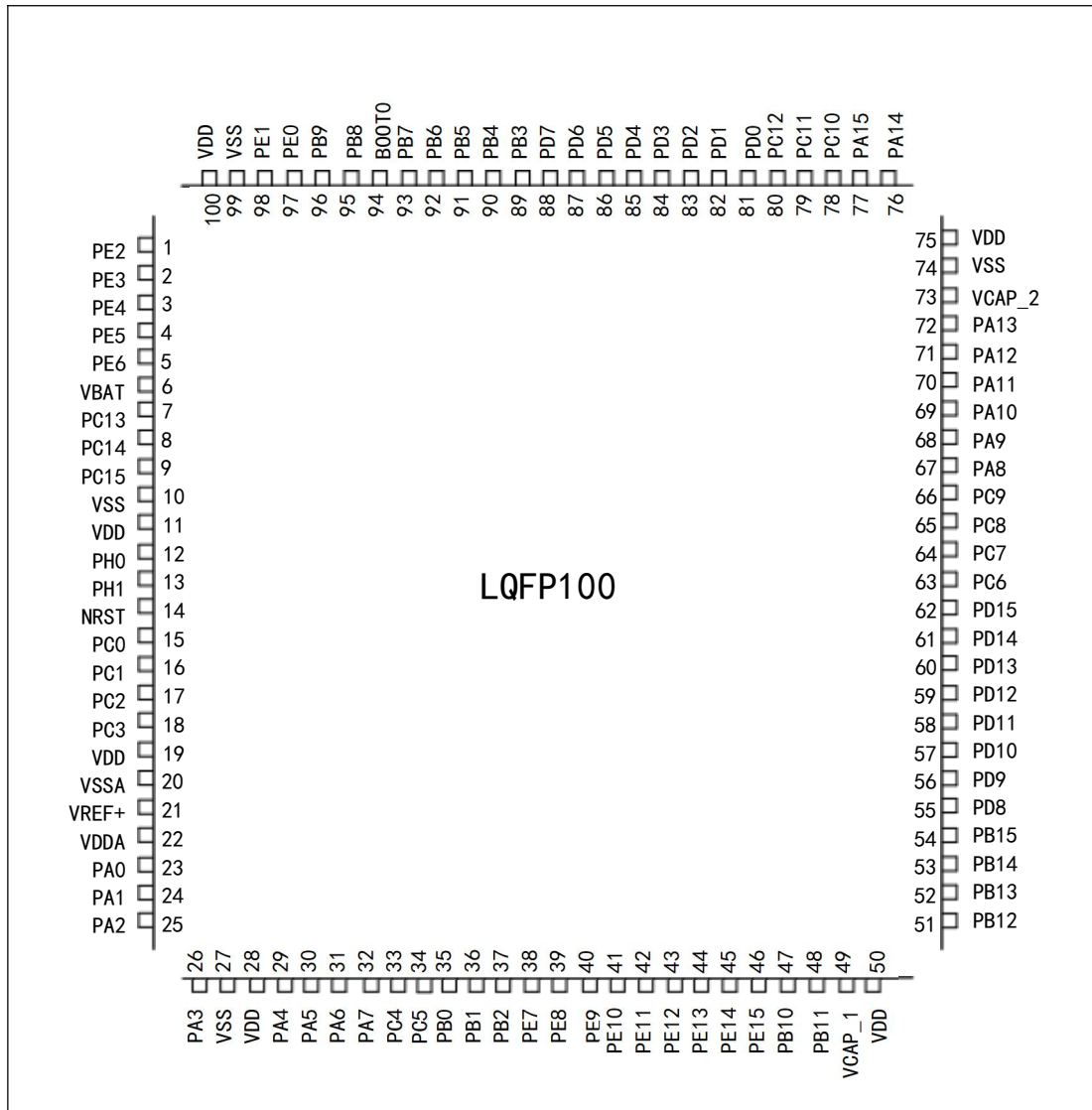
图 3 TLX32F407xG 系列 LQFP100 引脚分布图
