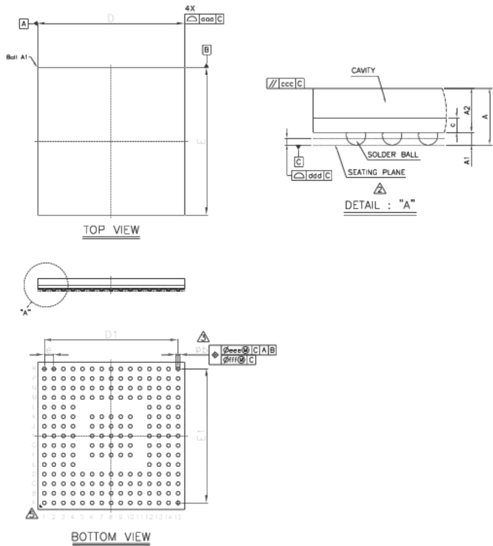
图 29 BGA176+25 封装图
