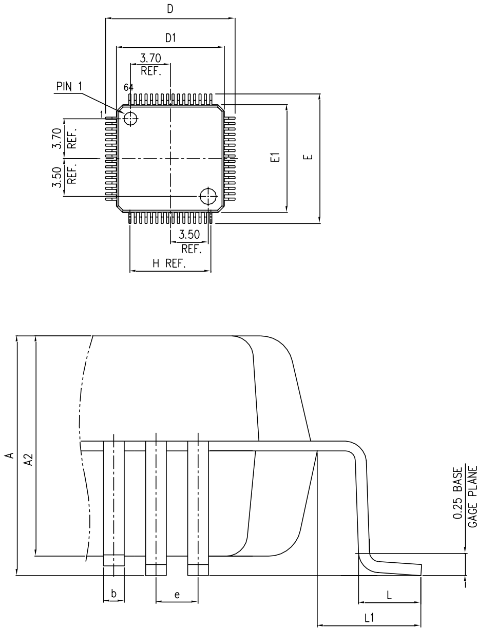
图 26 LQFP64 封装图
