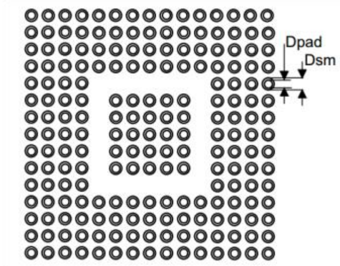
图 30 BGA176+25 -201-球，10 x10 mm，0.65mm 引脚间距，焊接 Layout 建议
