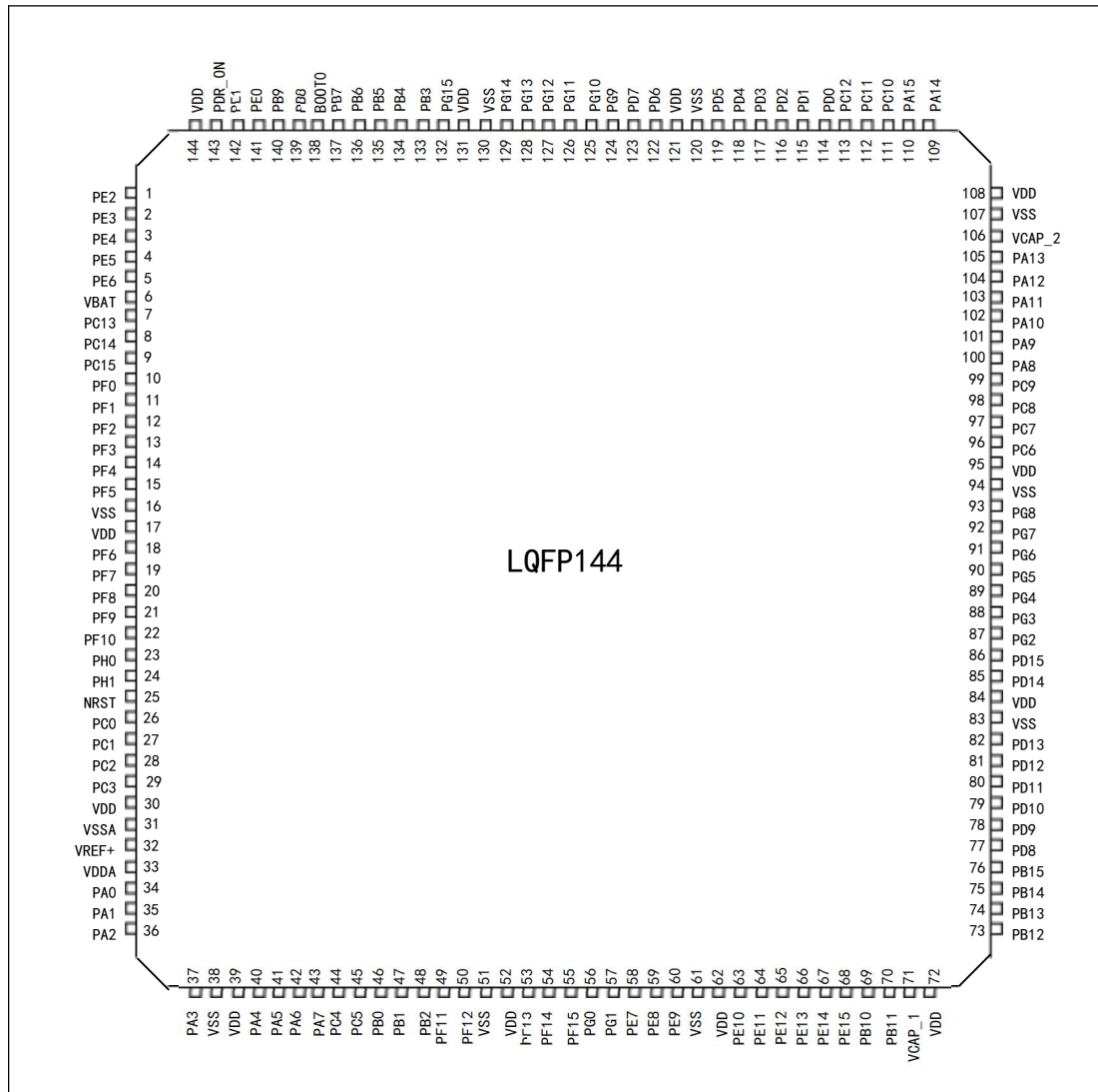
图 2 TLX32F407xG 系列 LQFP144 引脚分布图
