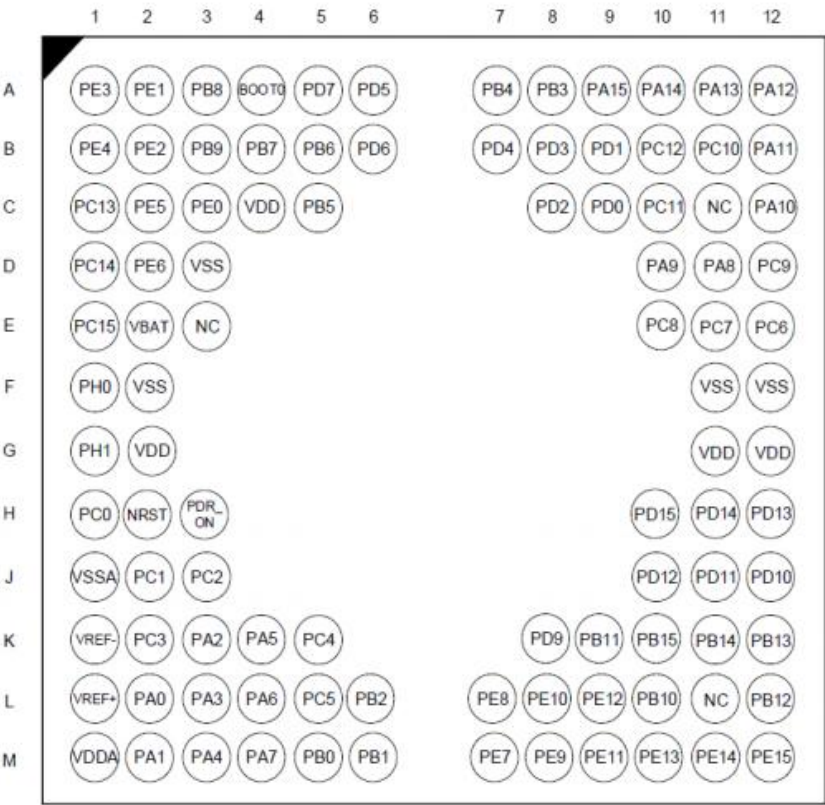
图 6 TLX32F407xG 系列 BGA100（7*7mm） 引脚分布图
