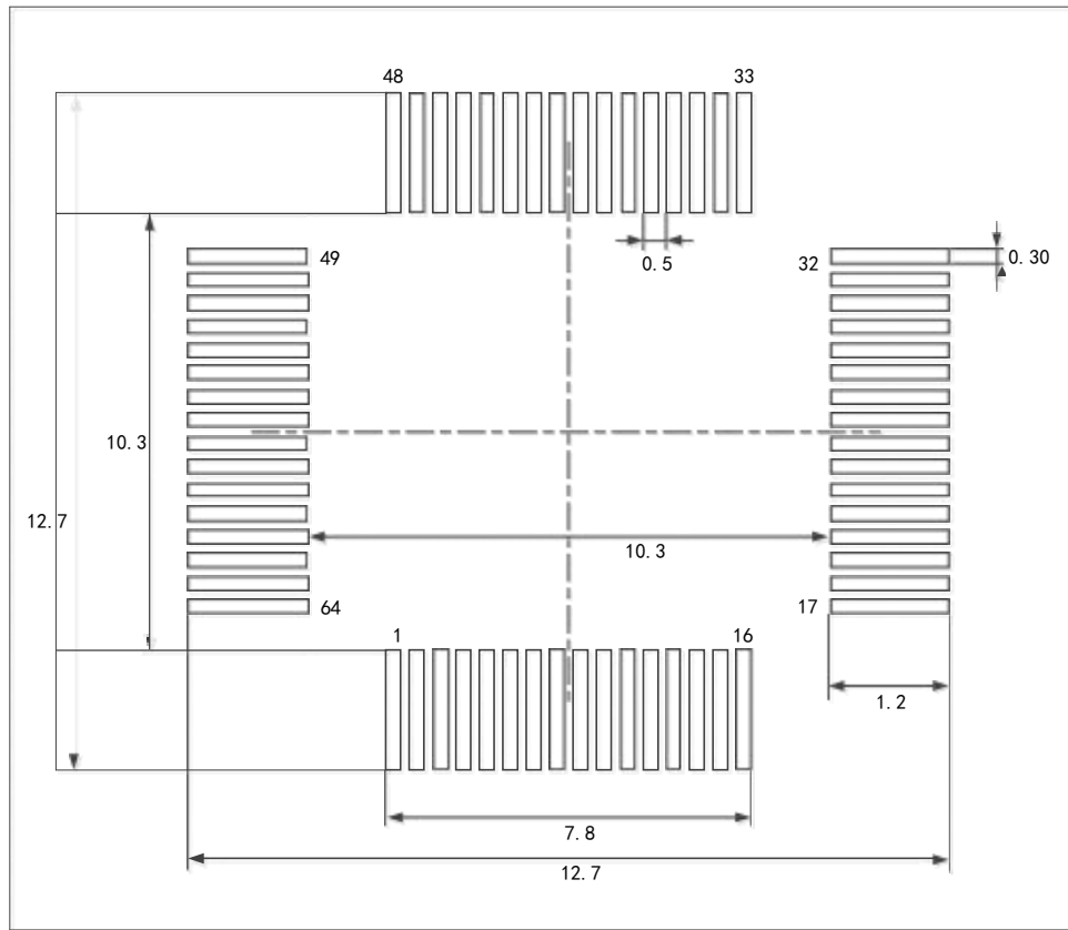
图 28 LQFP64 - 64 引脚，10 x 10mm 示意图
