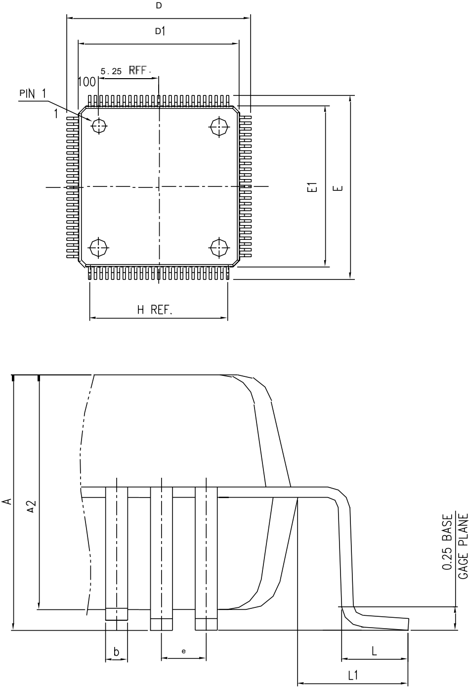
图 23 LQFP100 封装图
