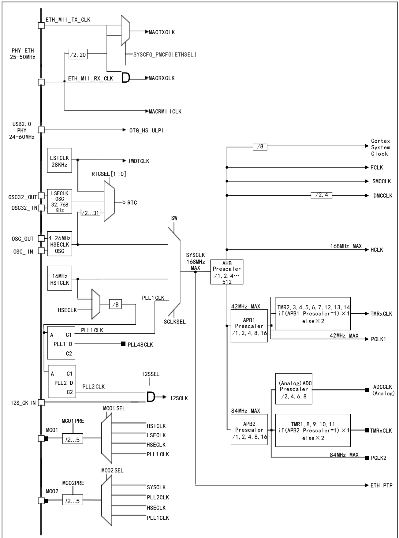
图 7 TLX32F407xG 时钟树
