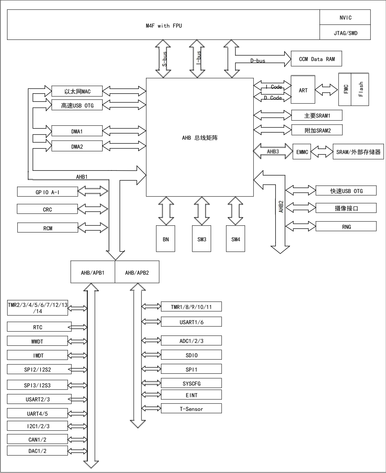
图 6 TLX32F407xG 系统框图
