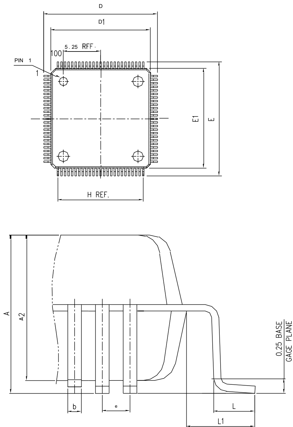
图 17 LQFP100 封装图
