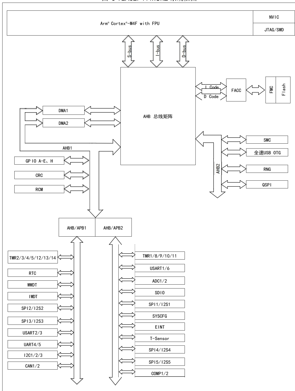
图 5 TLX32F411xCxE 系统框图
