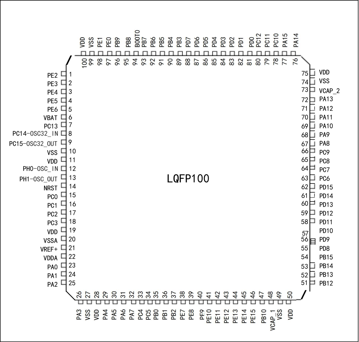
图 1 TLX32F411xCxE 系列 LQFP100 引脚分布图
