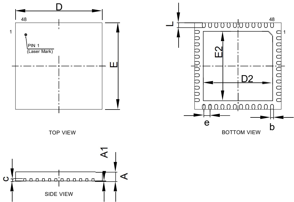
图 26 QFN48 封装图
