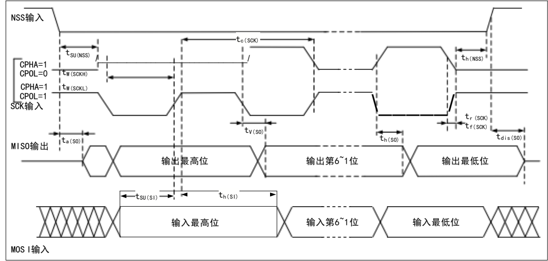
图 15 SPI 时序图—从模式和 CPHA=1
