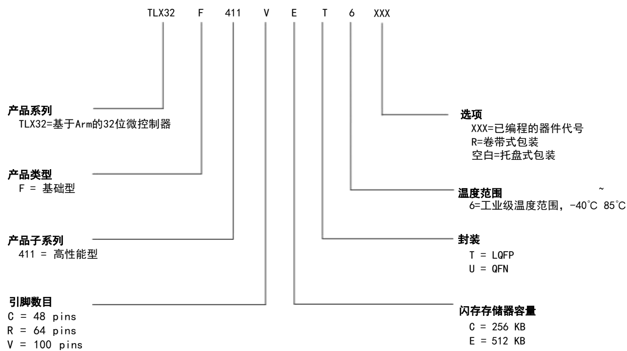
图 31 TLX32F411xCxE 系列订货信息图
