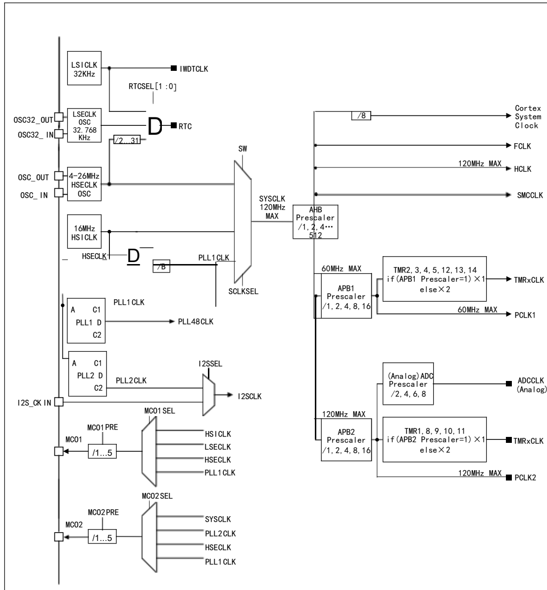
图 6 TLX32F411xCxE 时钟树
