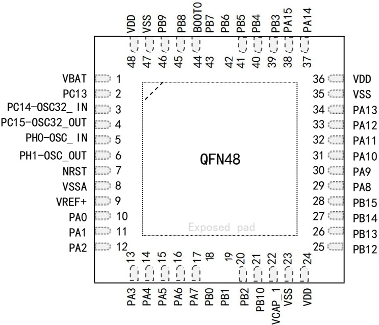
图 4 TLX32F411xCxE 系列 QFN48 引脚分布图
