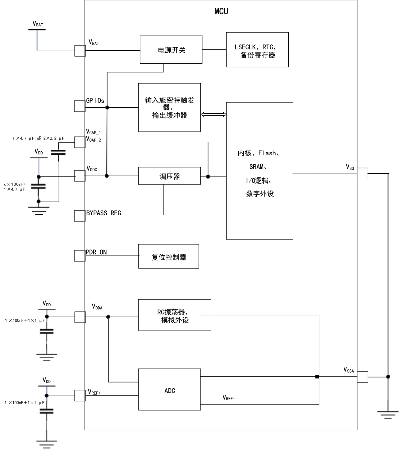
图 7 电源方案
