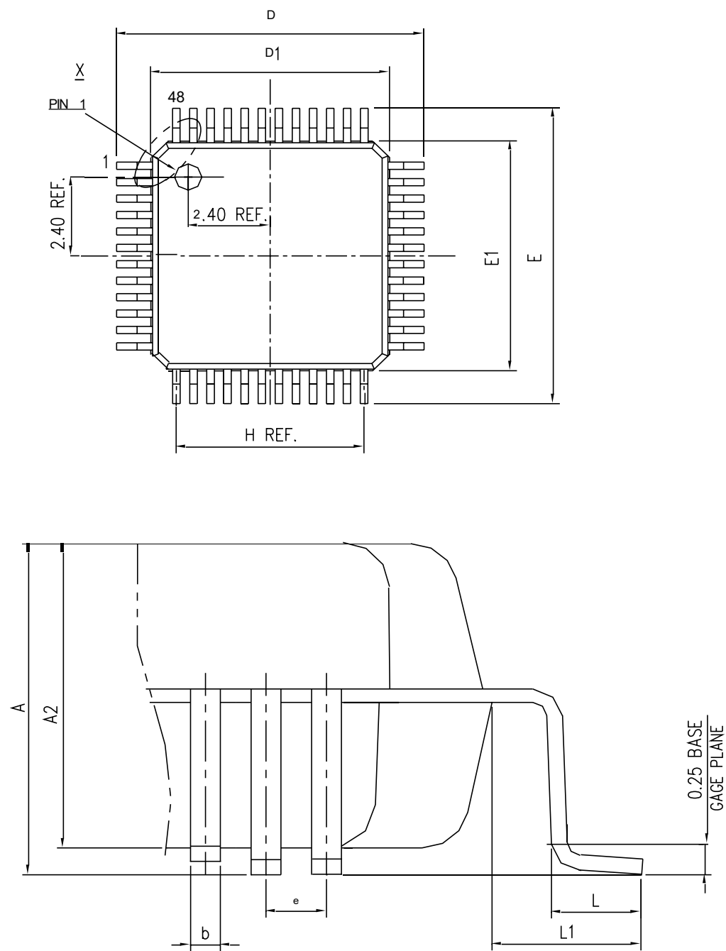
图 23 LQFP48 封装图
