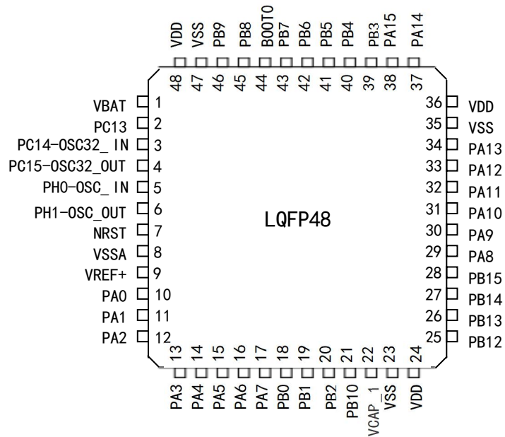
图 3 TLX32F411xCxE 系列 LQFP48 引脚分布图
