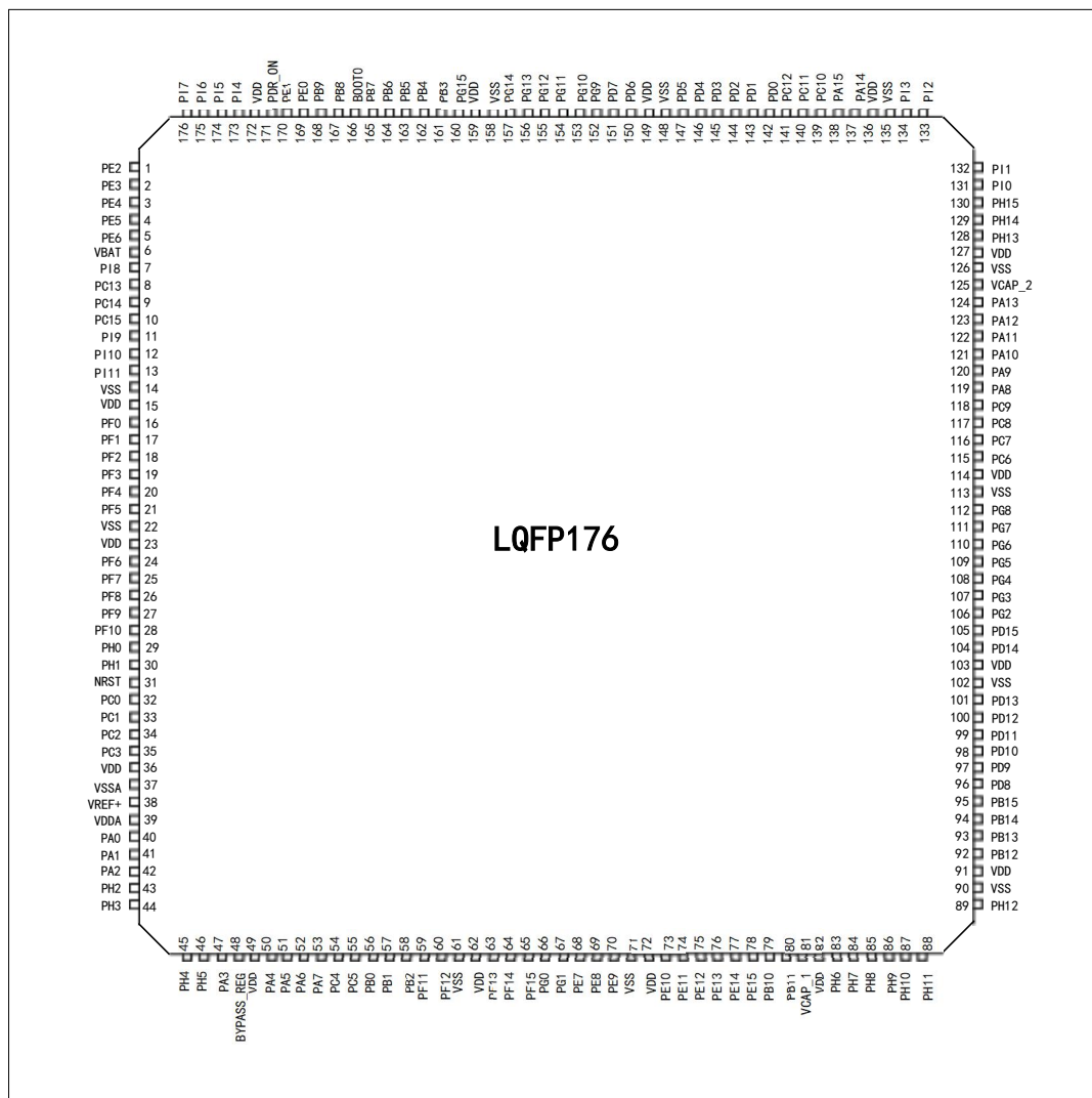
图 1 TLX32H407xGT6 系列 LQFP176 引脚分布图
