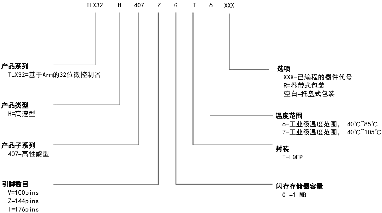
图 29 TLX32H407xGT6 系列订货信息图
