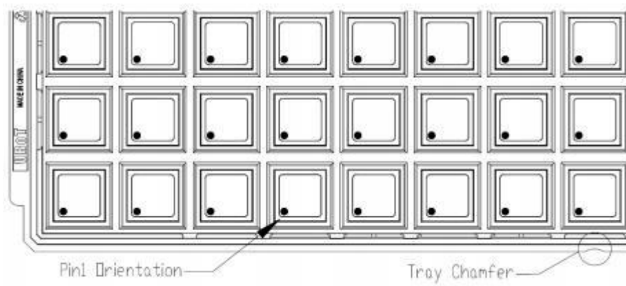
图 28 托盘包装示意图
