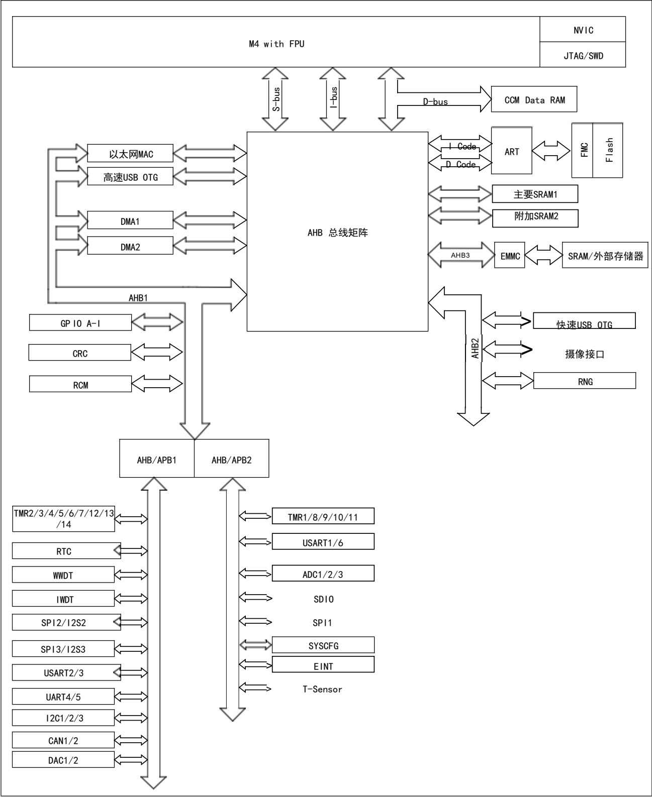
图 4 TLX32H407xGT6 系统框图
