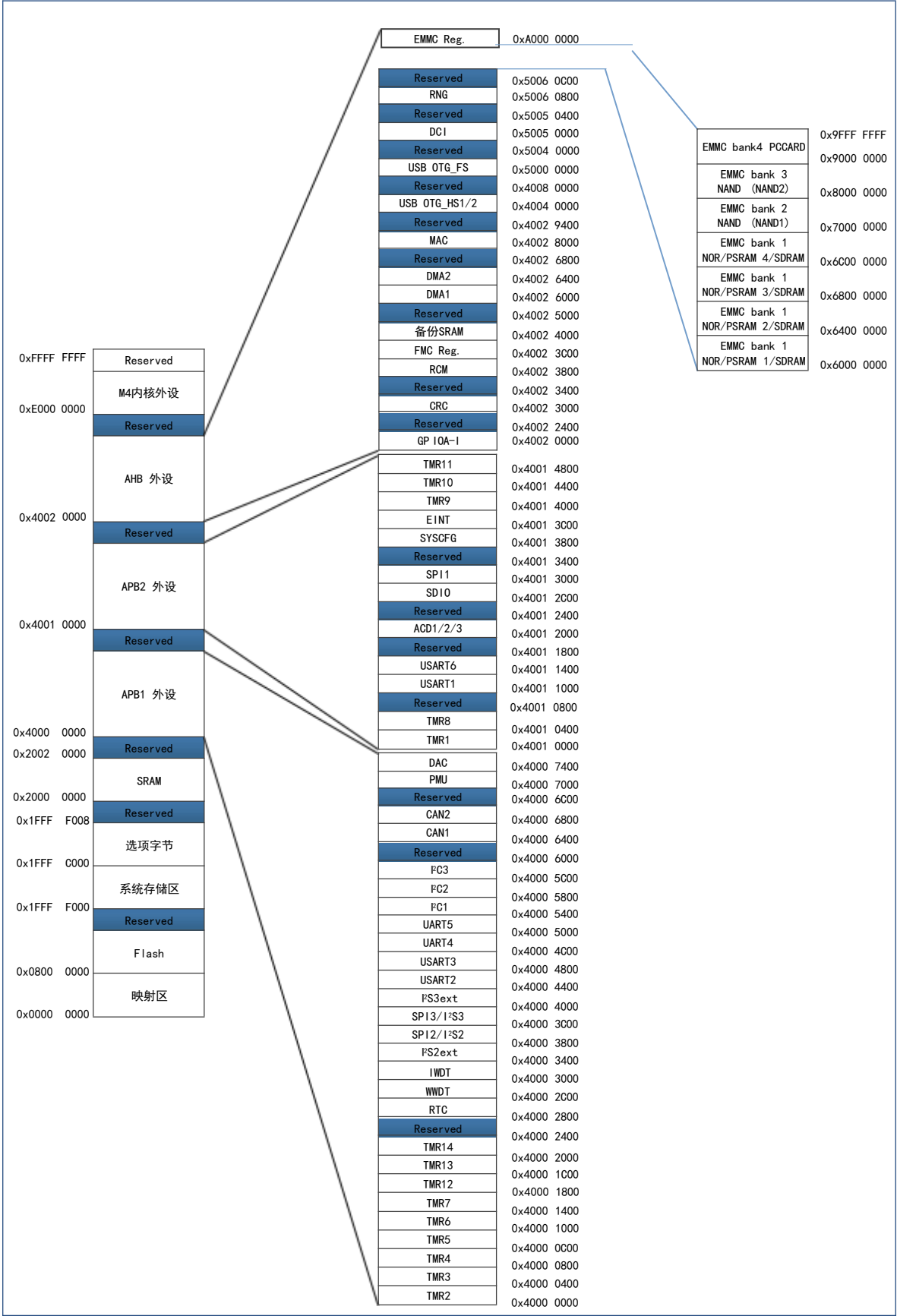
图 5 TLX32H407xGT6 系列地址映射图
