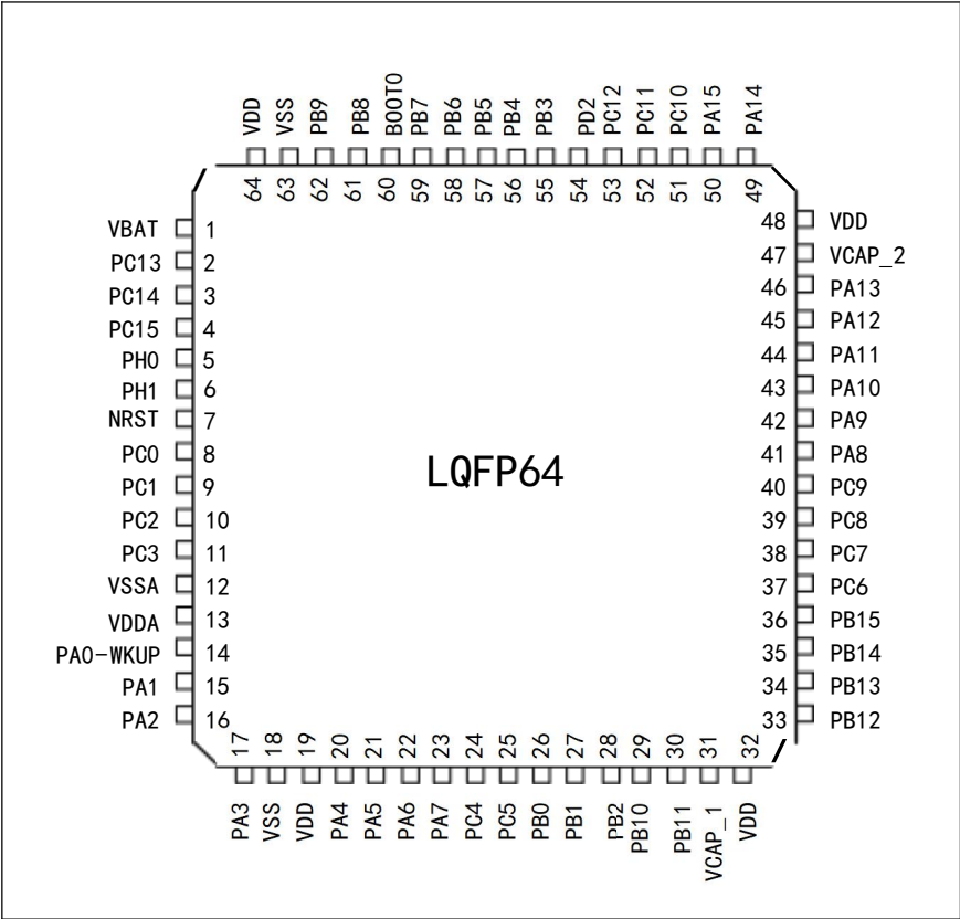
图 3 TLX32F405xG 407xExG 系列 LQFP64 引脚分布图
