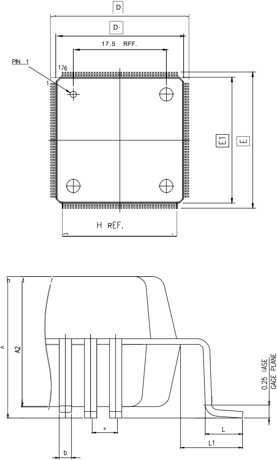
图 16 LQFP176 封装图
