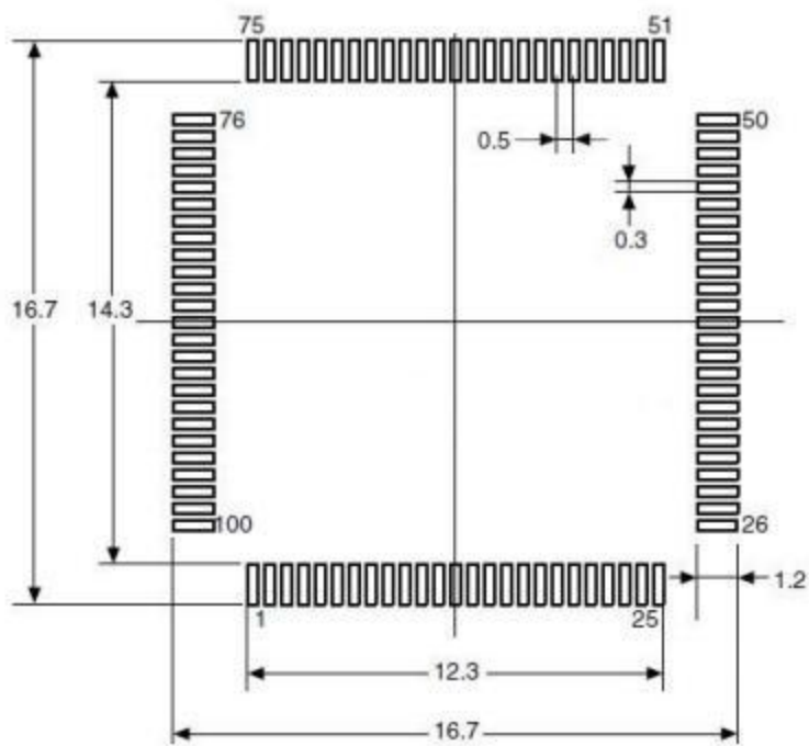
图 23 LQFP100 – 100 引脚，14 x 14mm 焊接 Layout 建议
