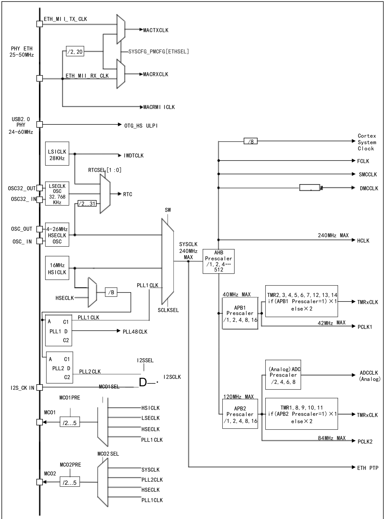
图 6 TLX32H407xGT6 时钟树
