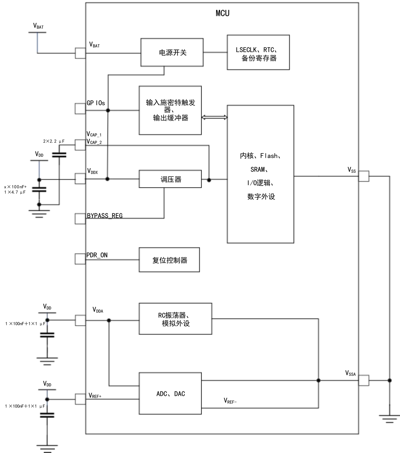
图 7 电源方案
