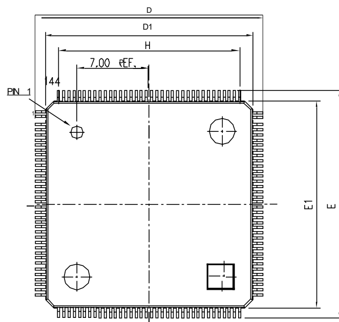
图 19 LQFP144 封装图
