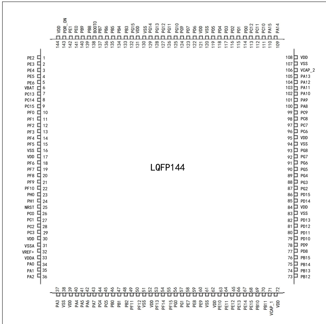
图 2 TLX32H407xGT6 系列 LQFP144 引脚分布图
