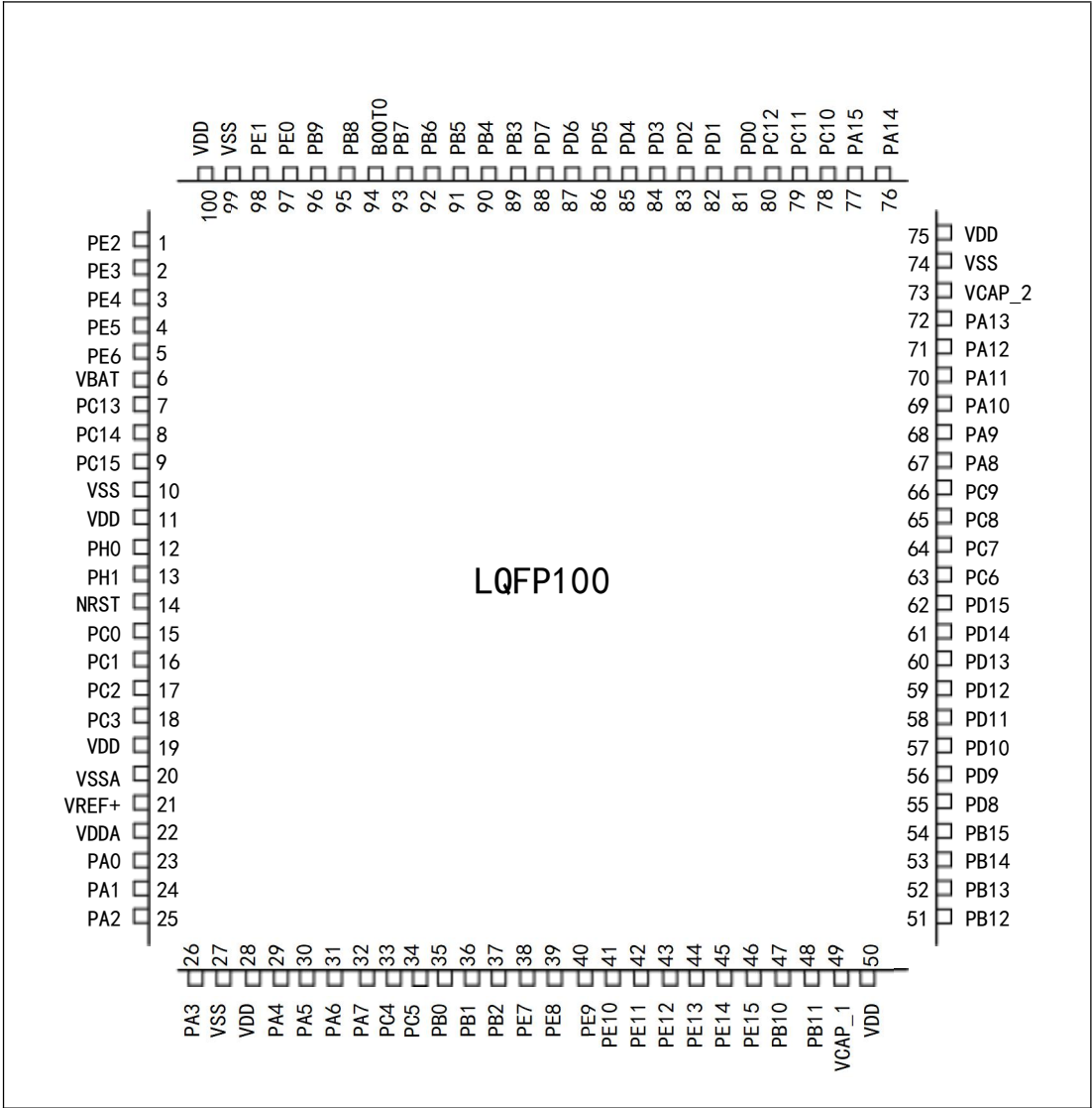
图 2 TLX32H407xGT6 系列 LQFP100 引脚分布图
