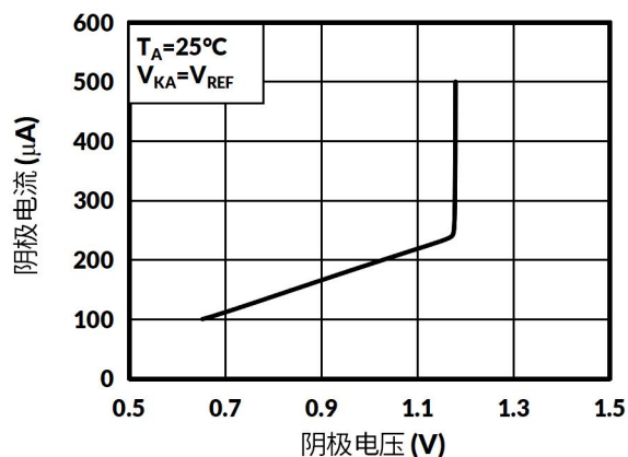
图 4. 阴极电流与阴极电压的关系
