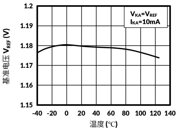
图 8. 基准电压与环境温度的关系
