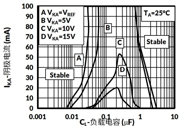
图 6. 阴极电流与负载电容的关系
