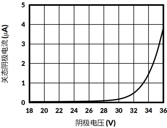
图 10. 阴极电压与关态阴极电流的关系
