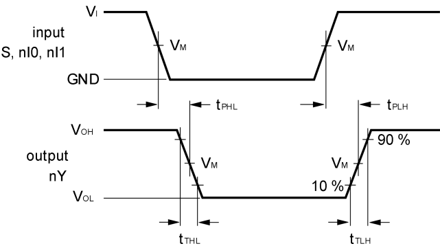
图 1. 输入 (nI0, nI1, S) 到输出 (nY) 的传播延迟
