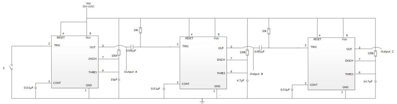
图 15 顺序计时器电路
