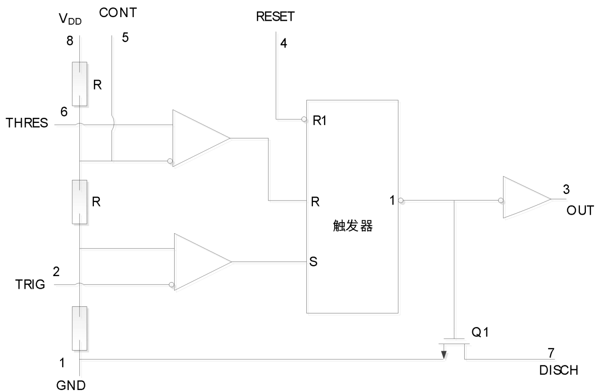
图 3 TLX555 芯片示意图
