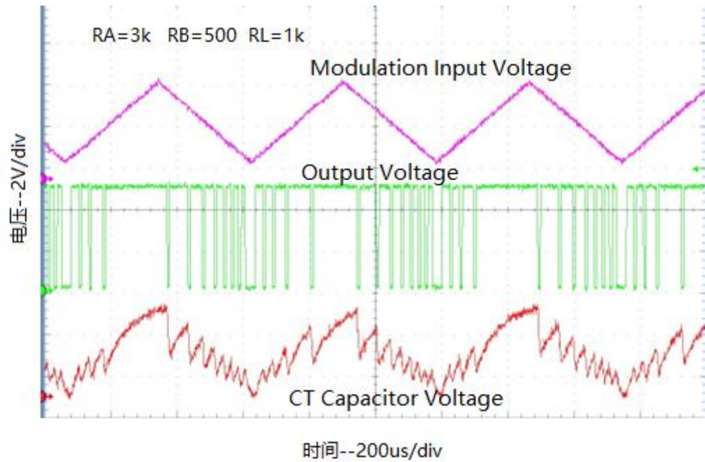
图 14 脉冲位置调制波形
