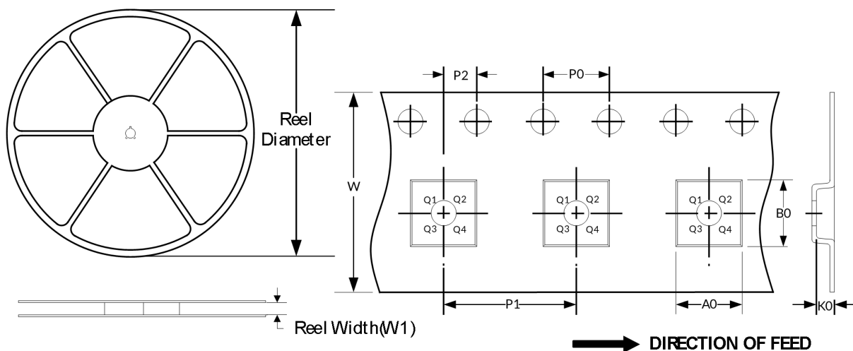
卷轴尺寸
