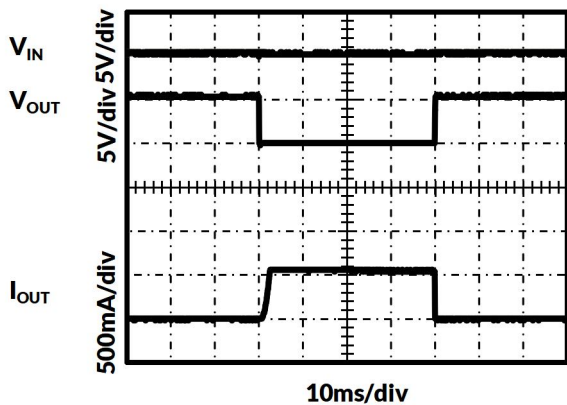
图 17. 空载短路
