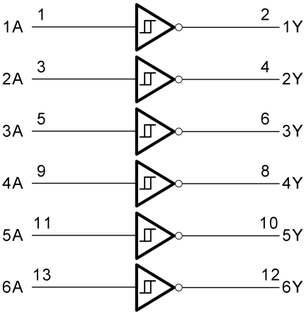
逻辑图示
