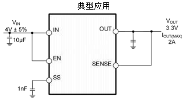
图 1 典型应用
