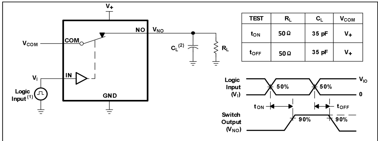
图 8.开启时间 ( t_{ON} ) 和关闭时间 ( t_{OFF} )
