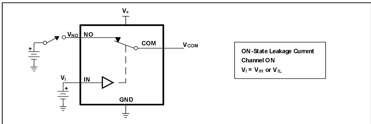
图 6. ON 状态漏电流 ( I_{COM(ON)} , I_{NO(ON)} )
