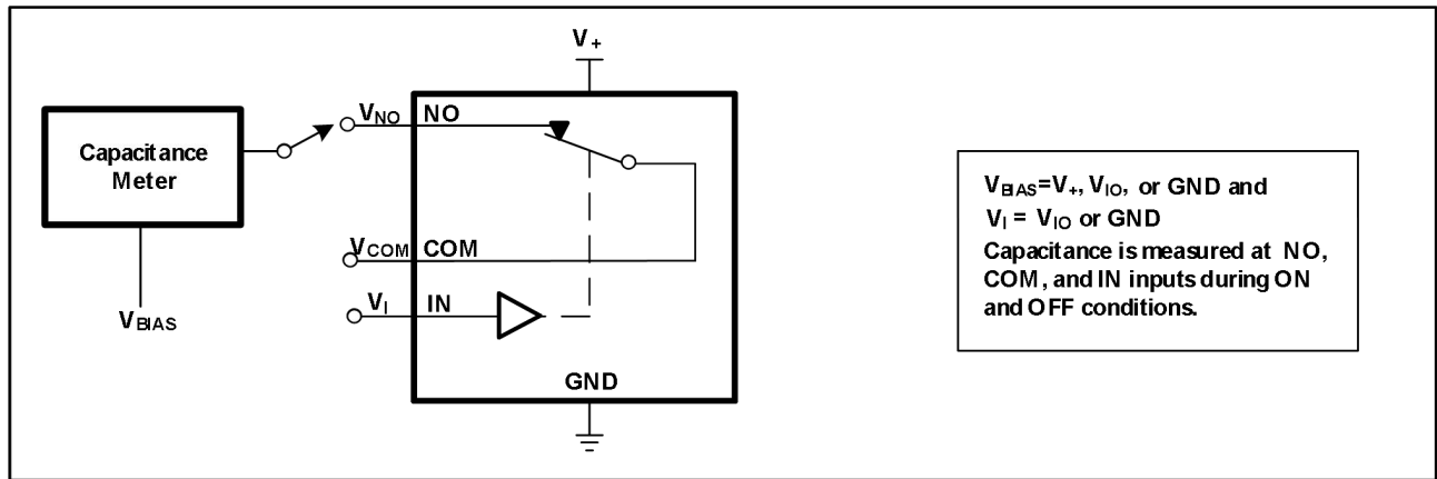
图 7.电容 ( C_I 、 C_{COM(OFF)} 、 C_{COM(ON)} 、 C_{NO(OFF)} 、 C_{NO(ON)} )
