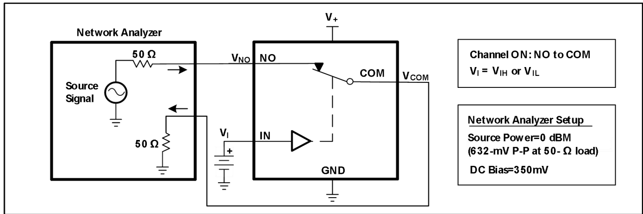
图 10. 带宽 (BW)
