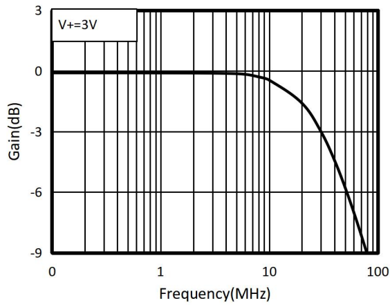
图 1. 带宽
