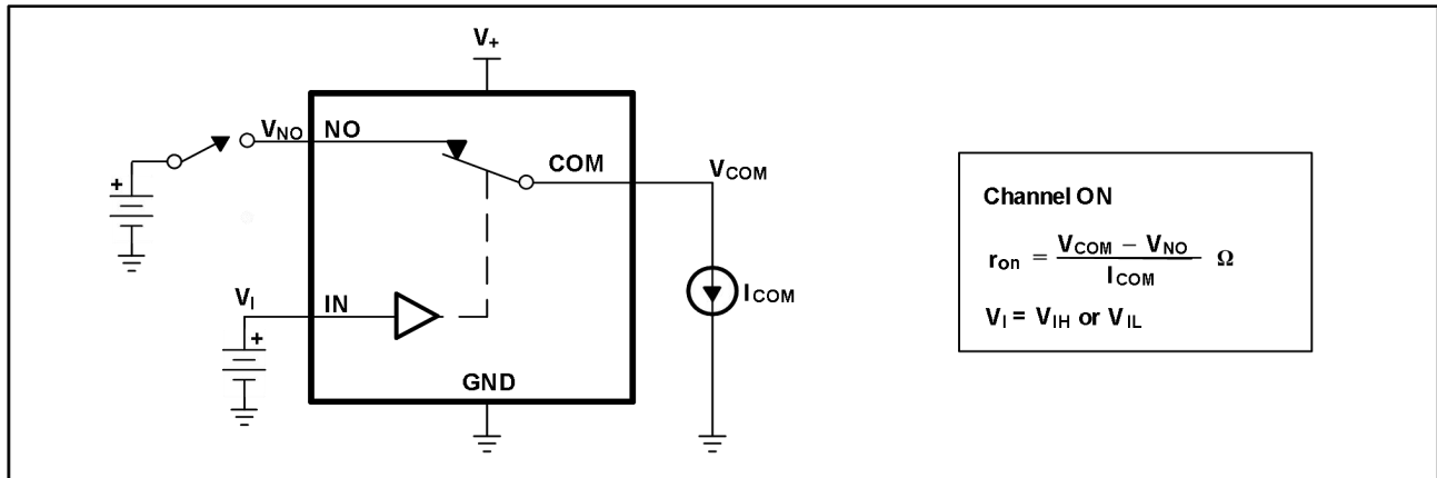
图 4. 导通电阻 ( r_{on} )
