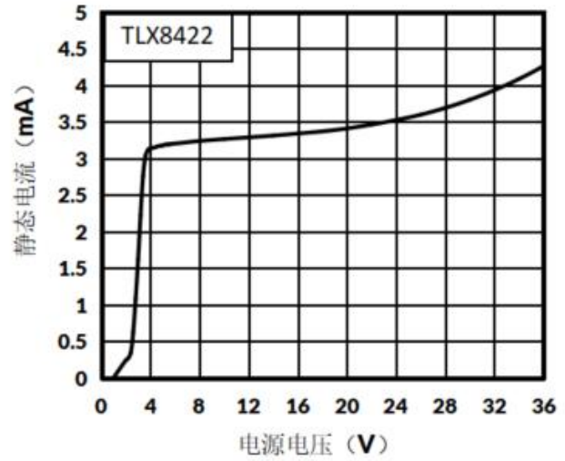
图 2. 电源电压与静态电流
