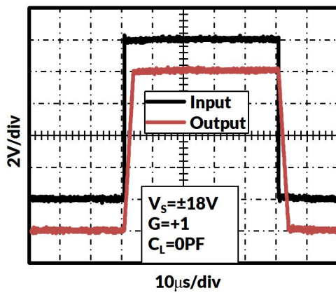
图 3. 大信号阶跃响应
