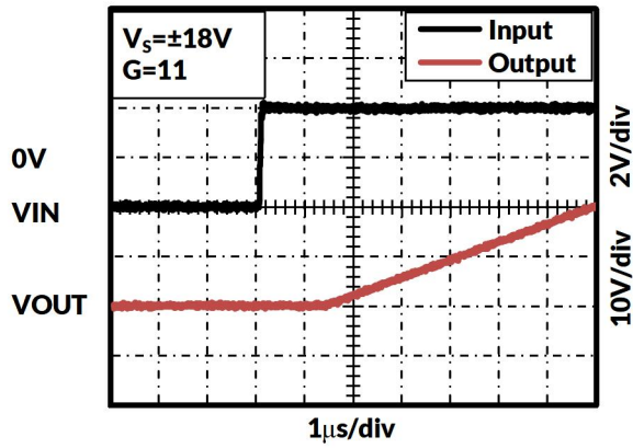
图 7. 正过压恢复
