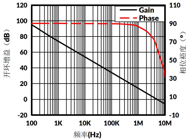
图 1. 开环增益和相位与频率的关系
