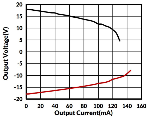
图 9. 输出电压摆幅与输出电流
