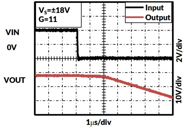
图 8. 负过压恢复
