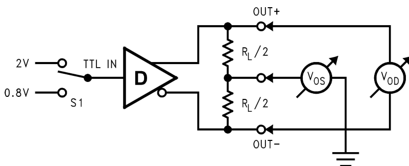
图 3 |VOD| 和 VOS 测试电路
