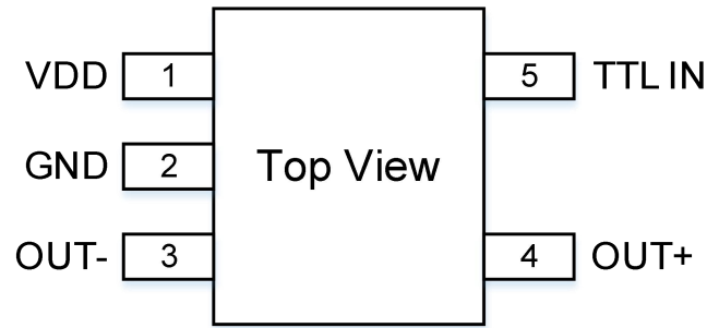
图 2. TLX90LV011 引脚配置
