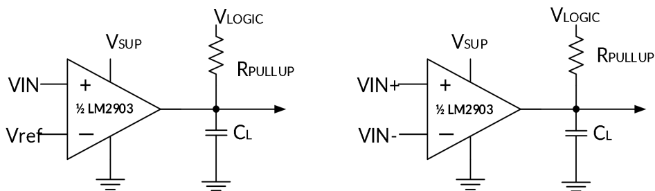
图 8. 单端和差分输入配置电路
