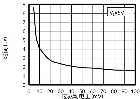
图 2. 响应时间与输入过驱动电压的关系 (正向跳变)
