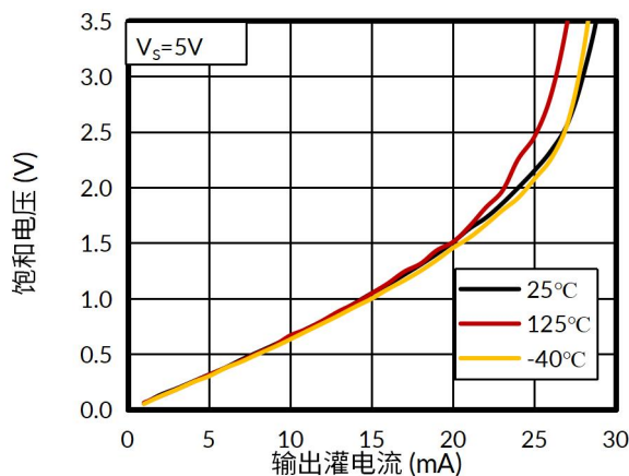
图 5. 饱和电压和输出灌电流的关系
