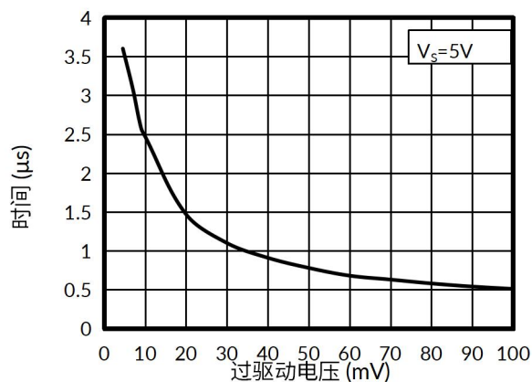
图 1. 响应时间与输入过驱动电压的关系 (负向跳变)
