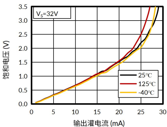
图 6. 饱和电压和输出灌电流的关系
