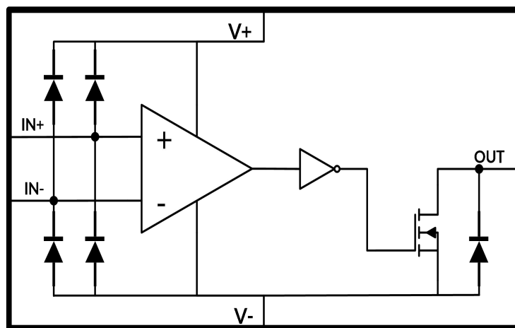
图 7. 功能框图
