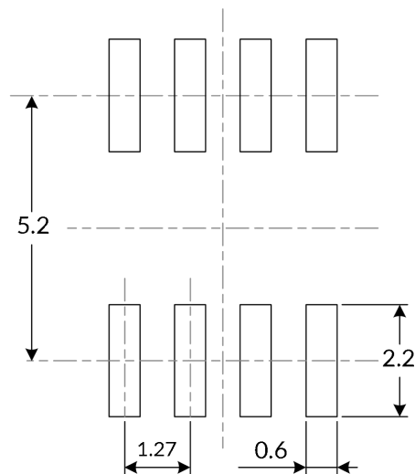
推荐焊盘尺寸 (单位: 毫米)
