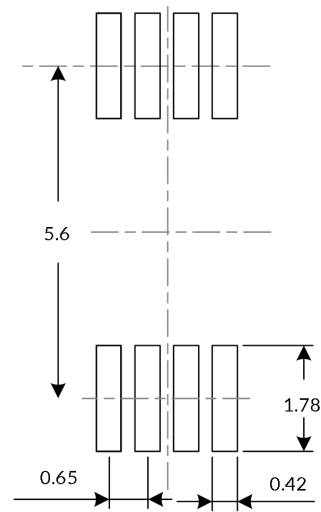
推荐焊盘尺寸 (单位: 毫米)
