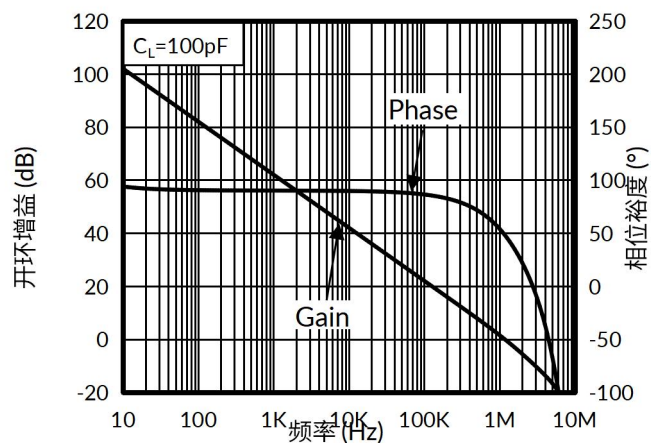
图 11. 开环增益和相位裕度与频率的关系
