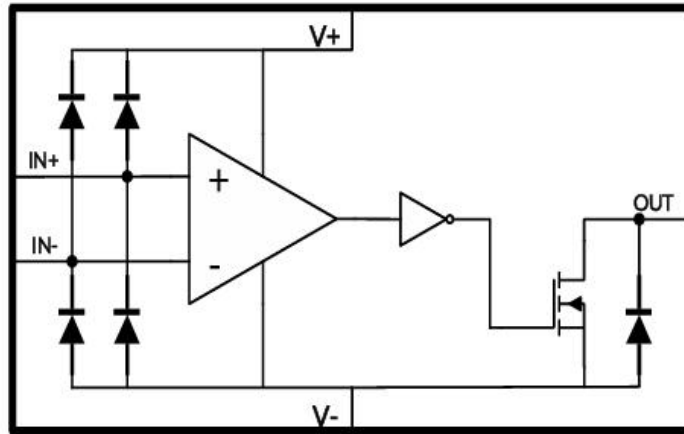
图 7. 功能框图
