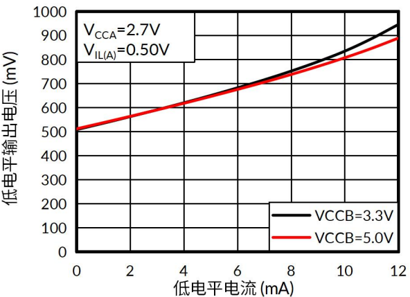
图 14. 低电平输出电压与低电平电流的关系
