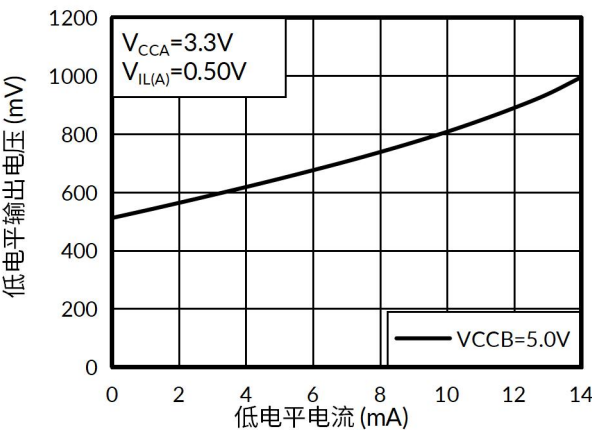
图 15. 低电平输出电压与低电平电流的关系
