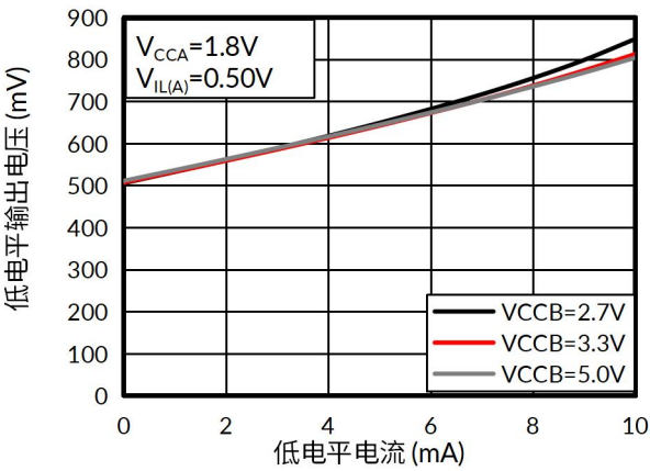
图 13. 低电平输出电压与低电平电流的关系
