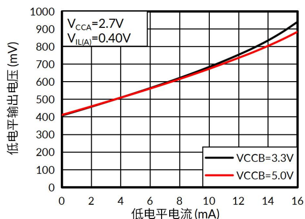
图 11. 低电平输出电压与低电平电流的关系
