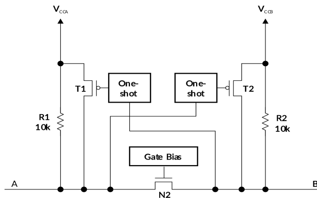
图 22. TLX0101 单元架构
