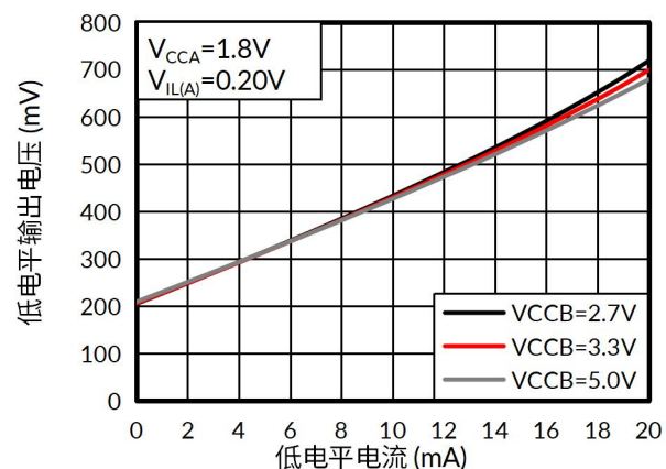
图 4. 低电平输出电压与低电平电流的关系
