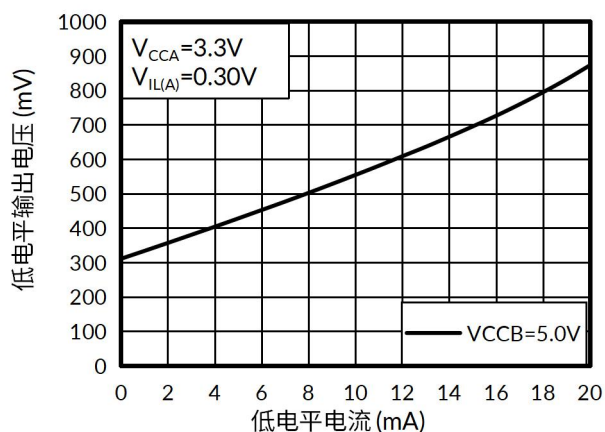
图 9. 低电平输出电压与低电平电流的关系
