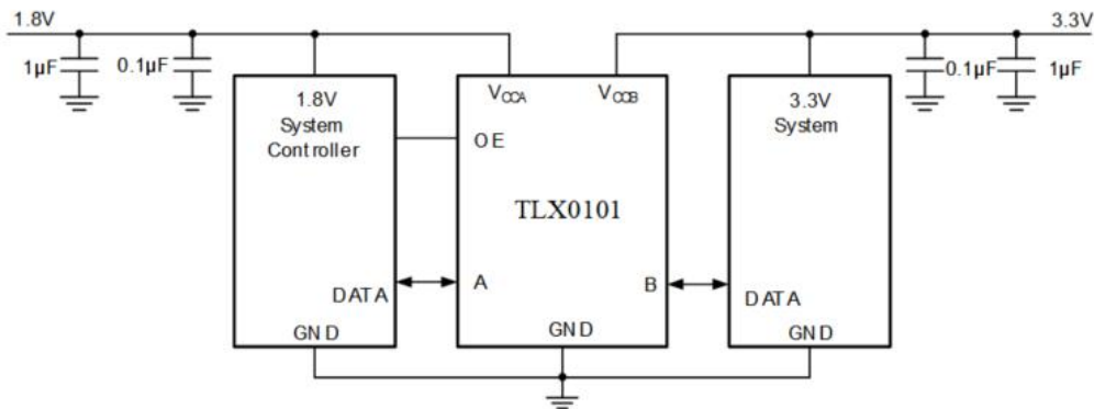
图 23. 典型应用电路
