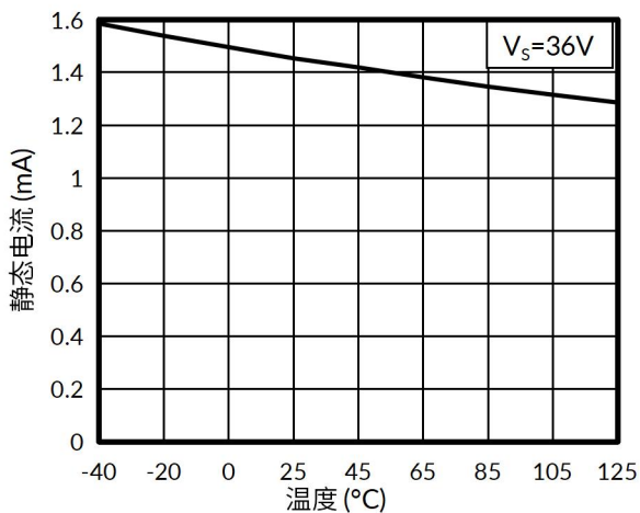
图 9. 静态电流与温度的关系
