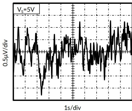
图 21. 0.1Hz~10Hz输入电压噪声
