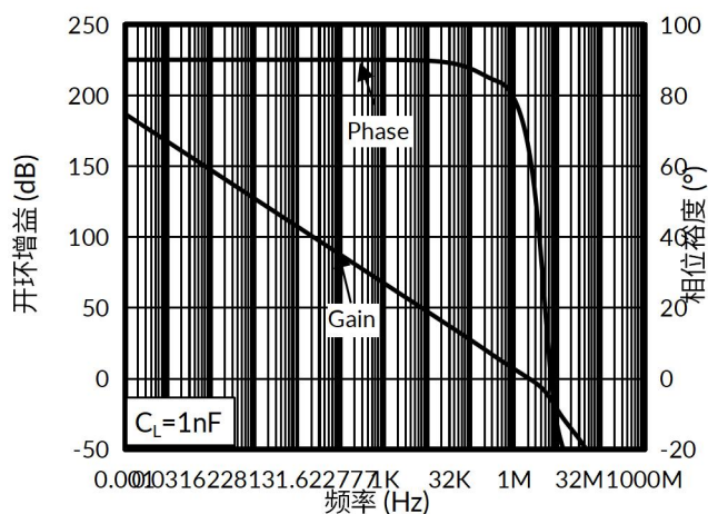
图 18. 开环增益和相位裕度与频率的关系
