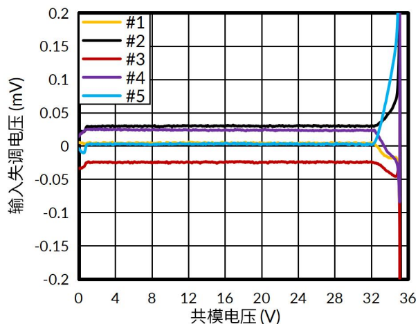
图 3. 输入失调电压与共模电压的关系
