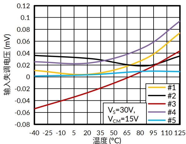
图 2. 输入失调电压与温度的关系
