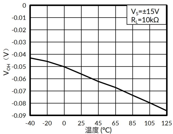
图 12. 输出距轨电压与温度的关系
