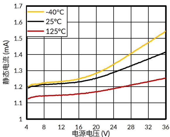
图 7. 静态电流与电源电压的关系
