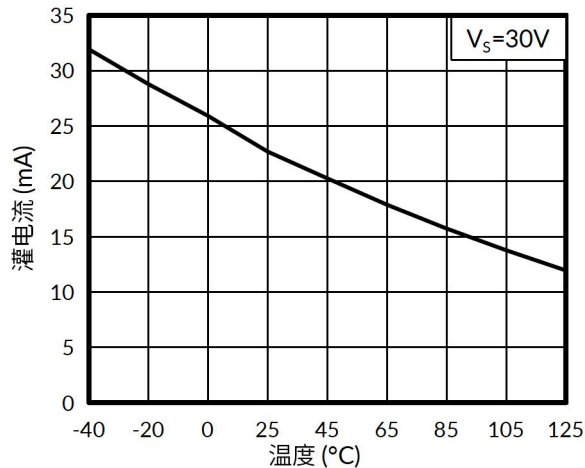
图 10. 灌电流与温度的关系
