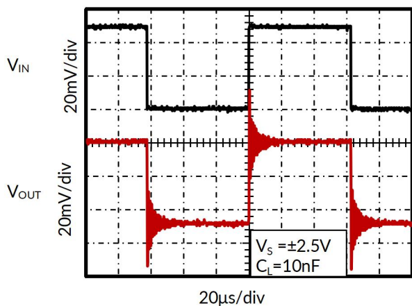
图 17. 小信号阶跃响应
