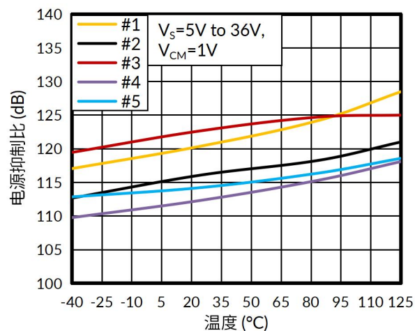
图 5. 电源抑制比与温度的关系
