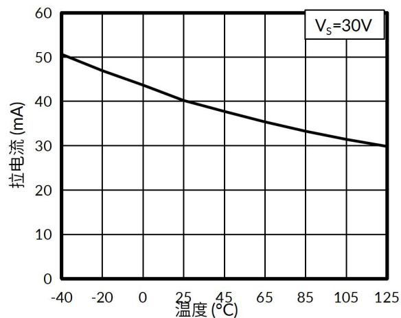
图 11. 拉电流与温度的关系
