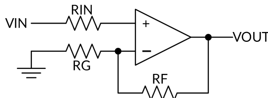
图 22. 同相放大器原理图
