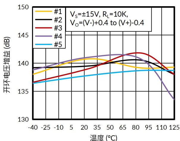
图 6. 开环电压增益与温度的关系
