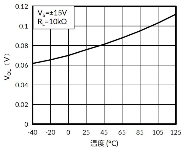
图 13. 输出距轨电压与温度的关系
