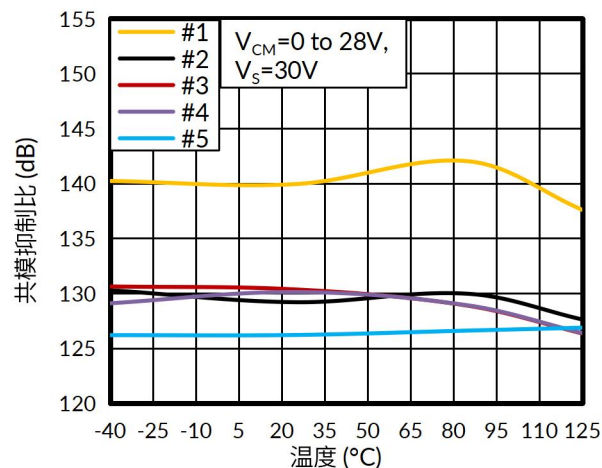
图 4. 共模抑制比与温度的关系
