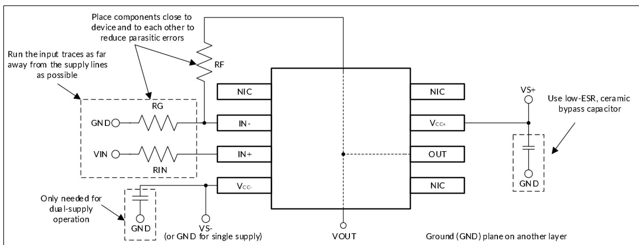
图 23. 运算放大器非反相配置的板级布局
