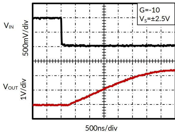
图 19. 反向过载恢复
