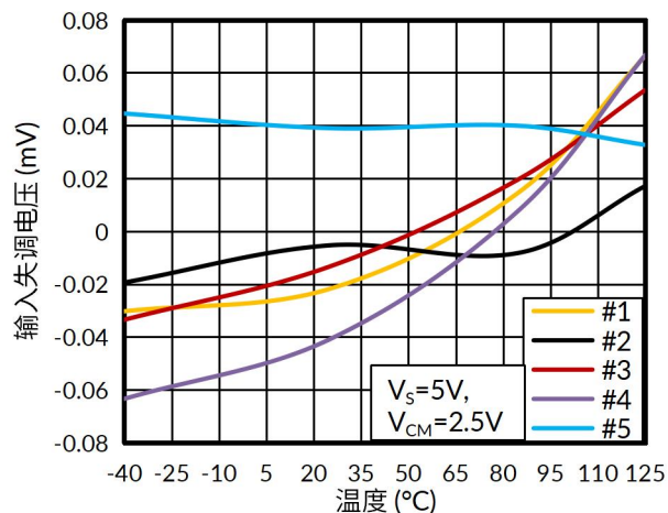
图 1. 输入失调电压与温度的关系
