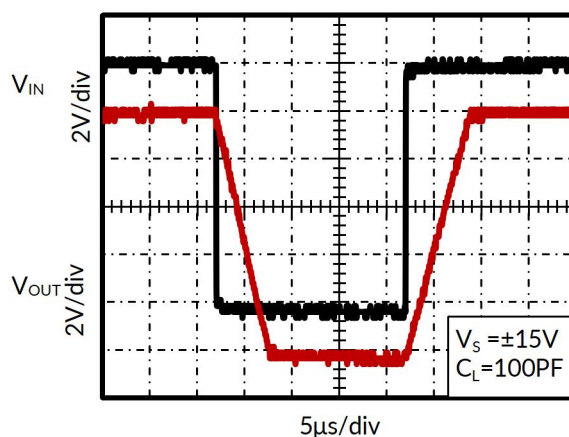
图 14. 大信号阶跃响应
