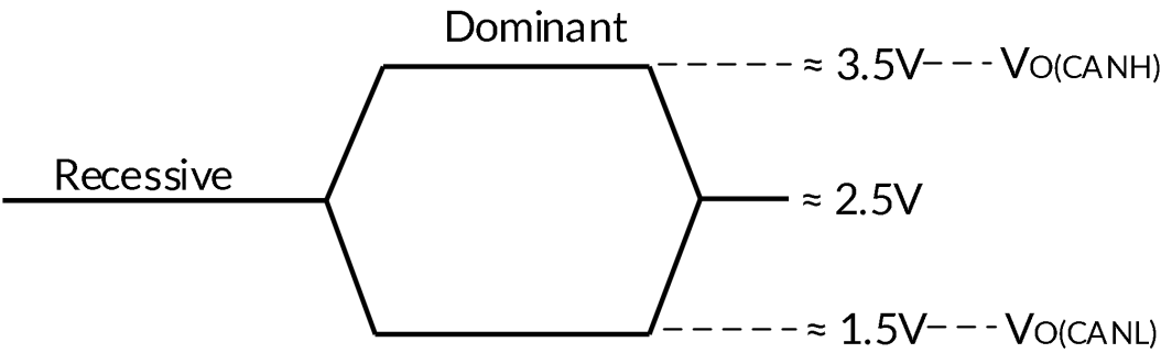
图 2. 总线逻辑状态电压定义
