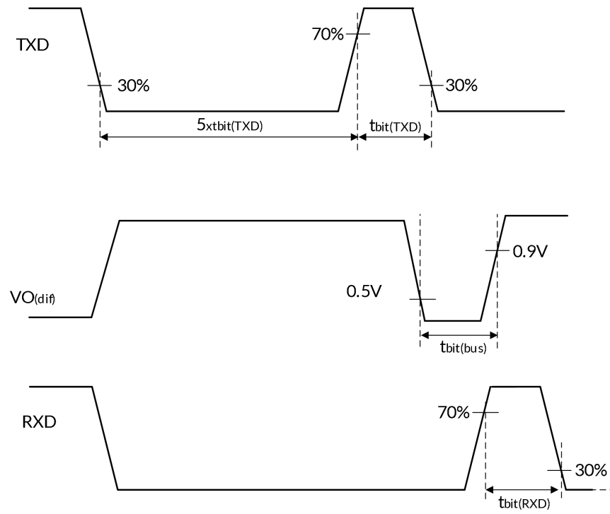
图 10. t_{\text{bit}}(\text{RXD}) 测试电路和波形
