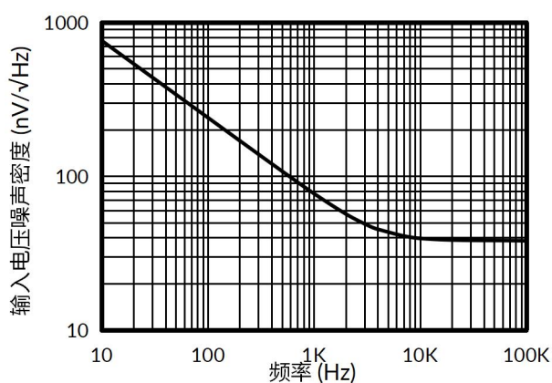
图 2. 输入电压噪声密度与频率的关系
