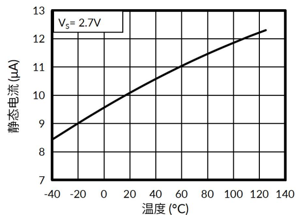
图 3. 静态电流与温度的关系
