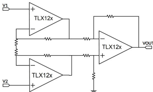
图 11. 仪表放大器
