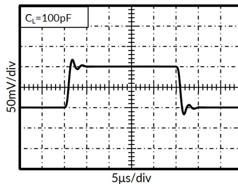
图 8. 小信号阶跃响应
