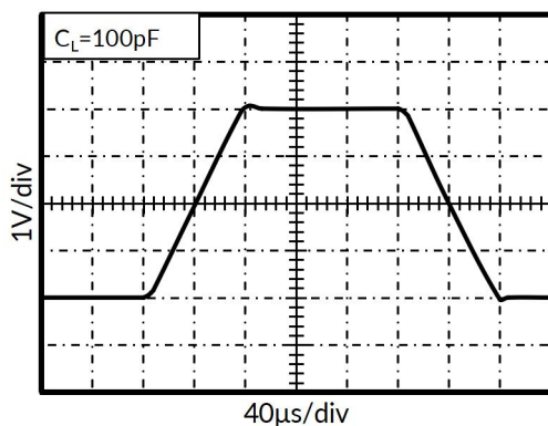
图 9. 大信号阶跃响应
