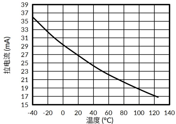
图 6. 拉电流与温度的关系
