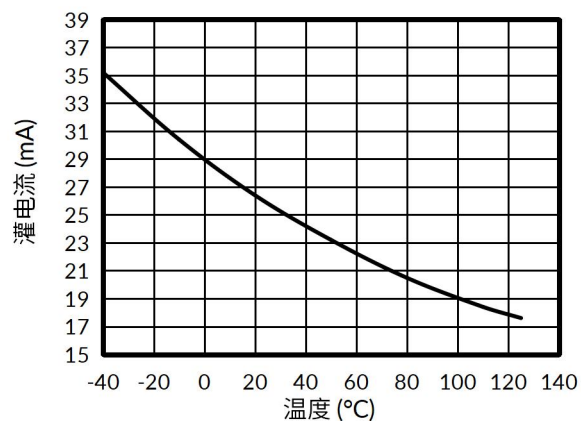
图 5. 灌电流与温度的关系
