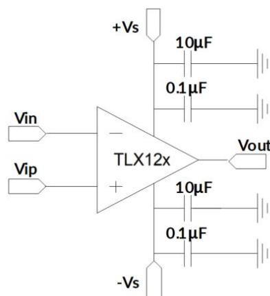
图 10. 带旁路电容器的放大器
