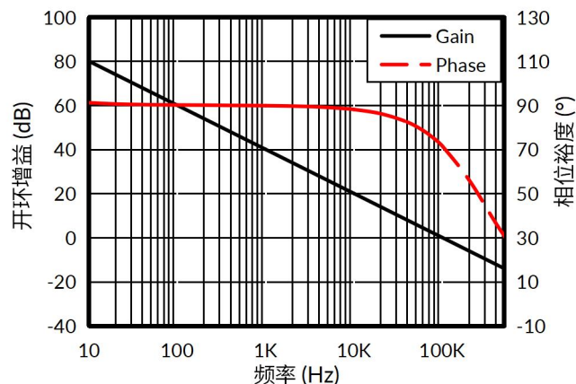
图 1. 开环增益和相位裕度与频率的关系
