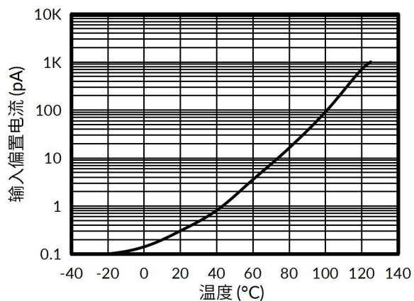
图 7. 输入偏置电流与温度的关系
