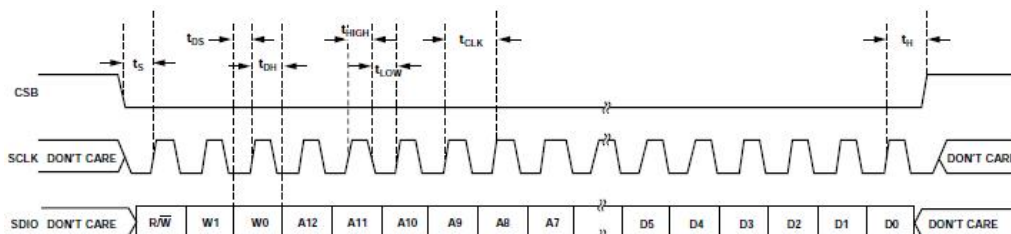
图 9. SPI 串行端口接口时序
