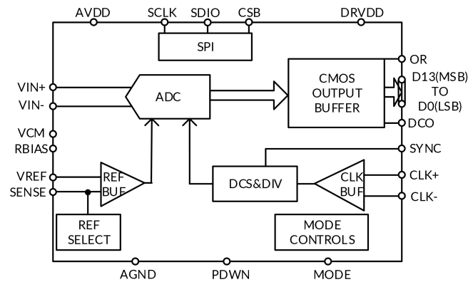
图 1. TLX1520系统框图
