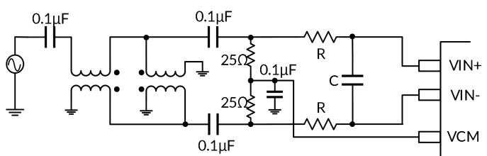
图 4. 差分双巴伦输入配置
