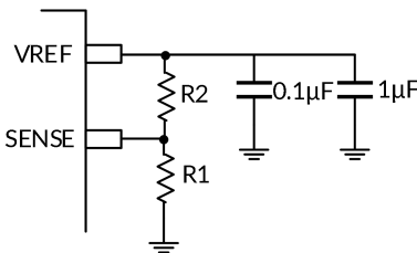
图 8. 可编程基准电压模式
