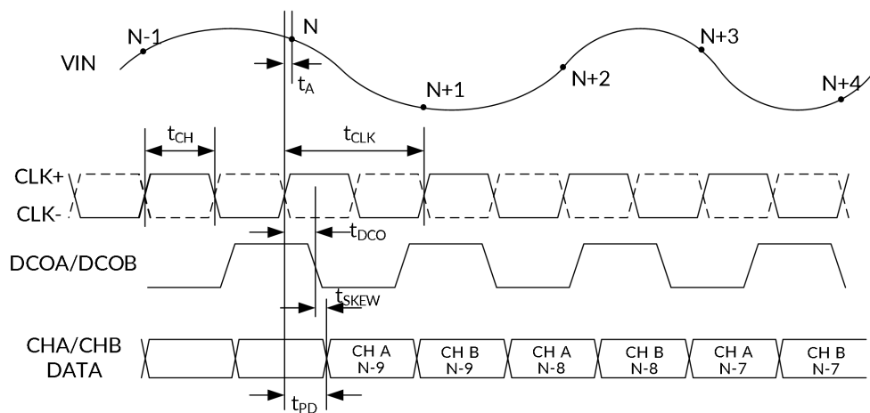
图 3. CMOS 交错输出模式数据输出时序
