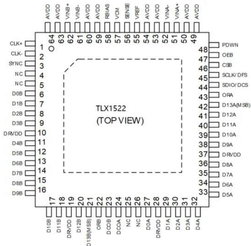
QFN9X9-64
