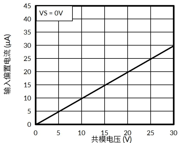
图 14. 输入偏置电流与共模电压的关系 (双输入，关断模式)
