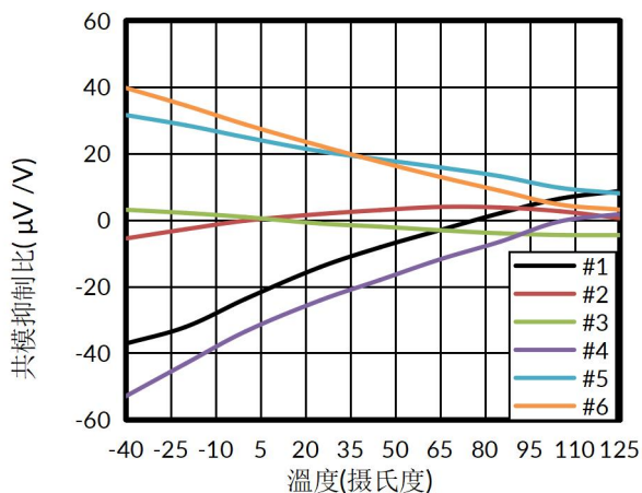
图 4. 共模抑制比与温度
