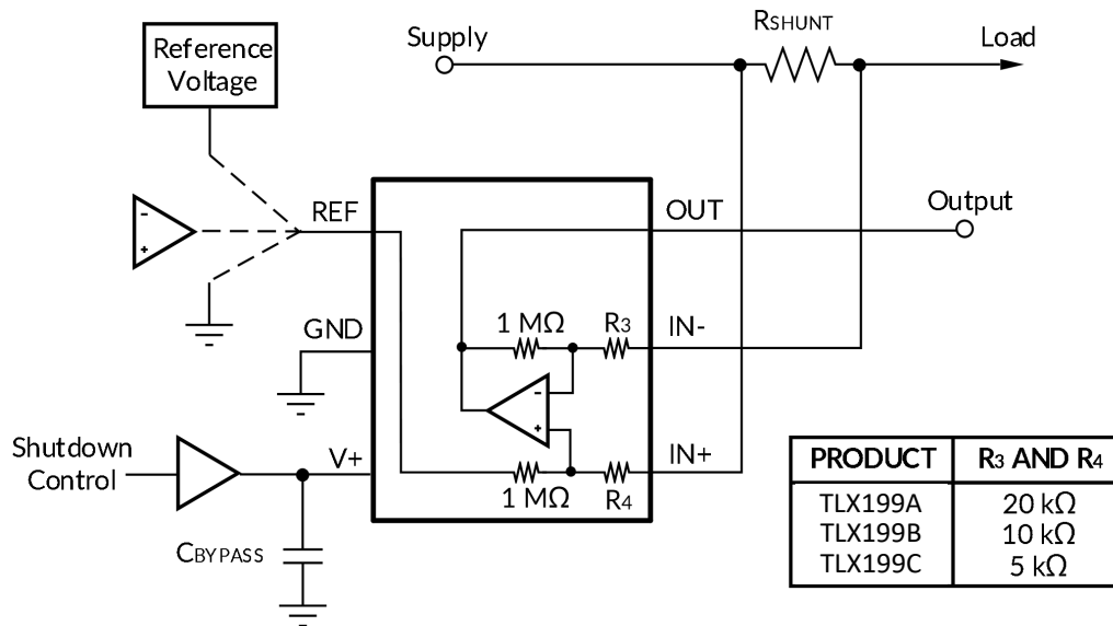
图 15. 关闭 TLX199 的基本电路 具有接地参考
