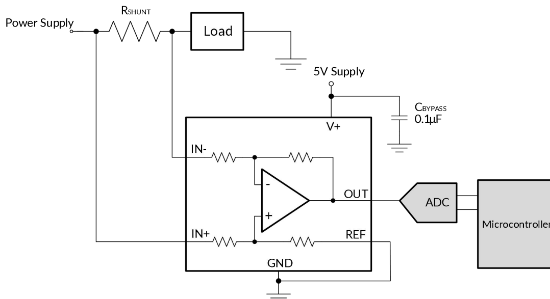
图 17. 典型应用
