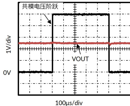
图 14. 共模电压瞬态响应
