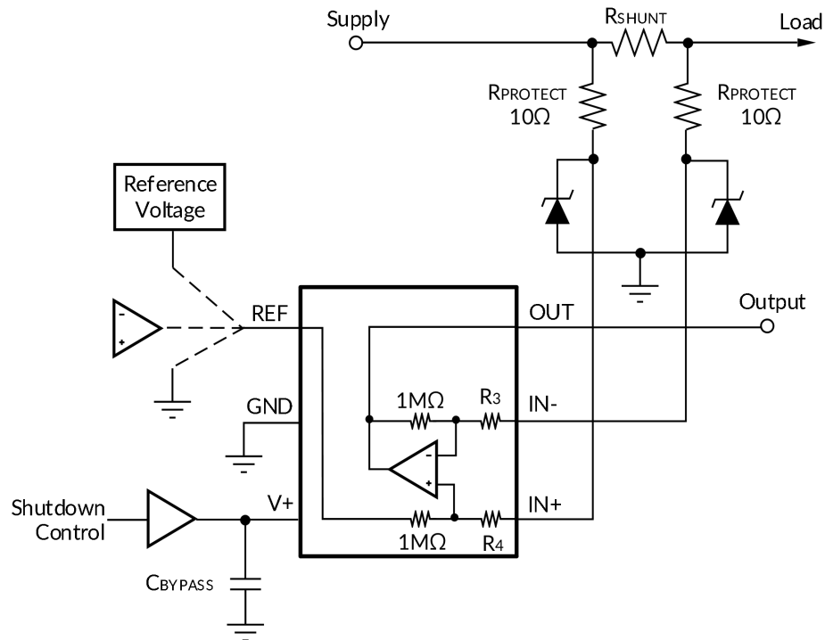
图 21. TLX199XP 采用双齐纳二极管的瞬态保护电路
