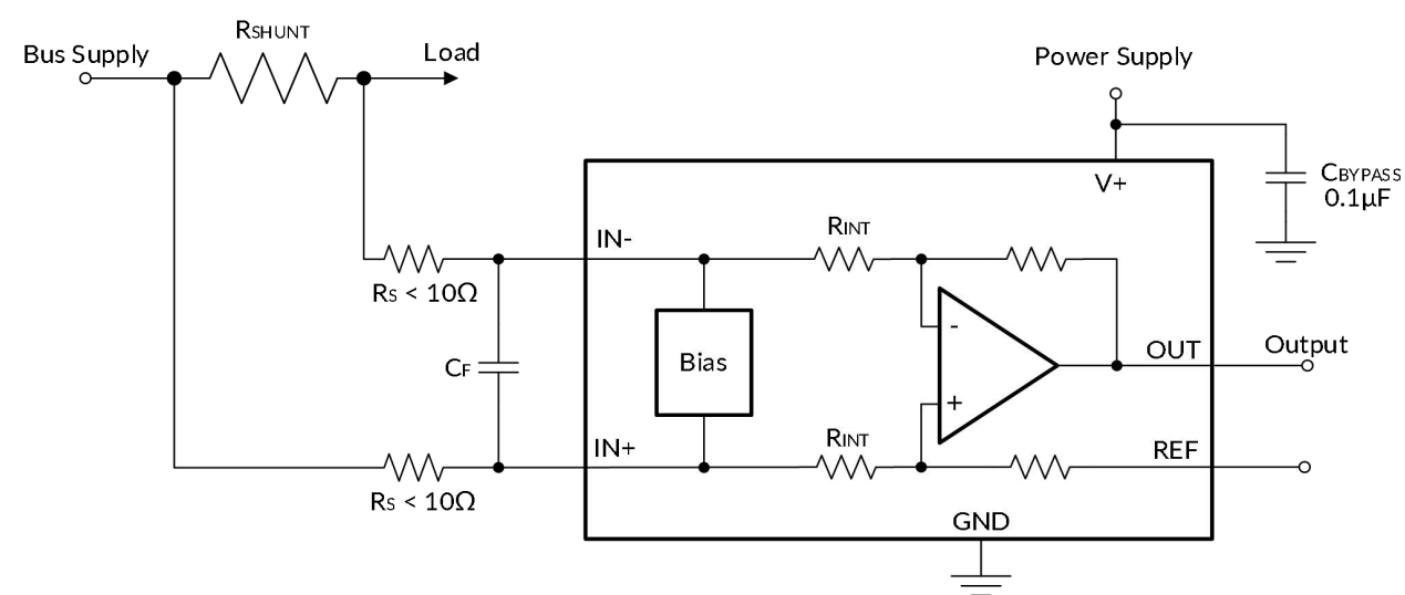
图 18. 输入引脚上的滤波
