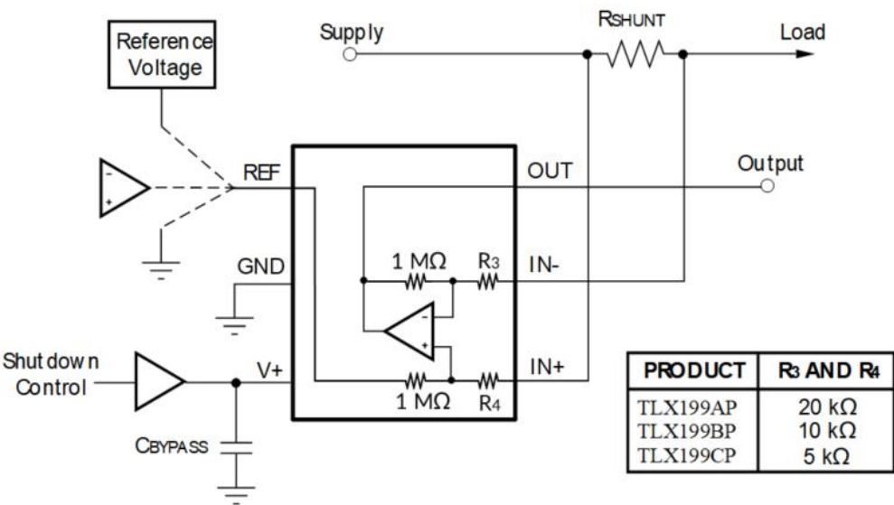
图 19. 含接地基准的 TLX199XP 关断电路
