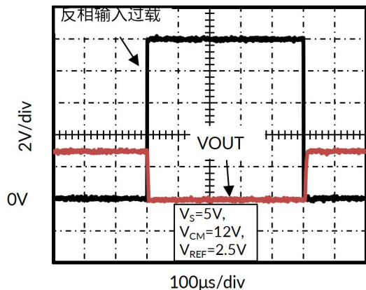
图 13. 反相差分输入过载
