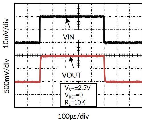
图 11. 阶跃响应 ( 20\text{mV}_{PP} 输入阶跃)
