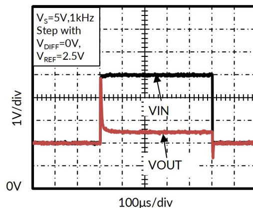
图 16. 掉电恢复
