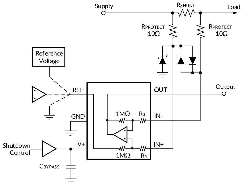
图 22. TLX199XP 采用瞬态吸收器件和输入钳位的瞬态保护电路
