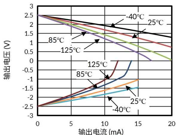
图 5. 输出电压与输出电流的关系
