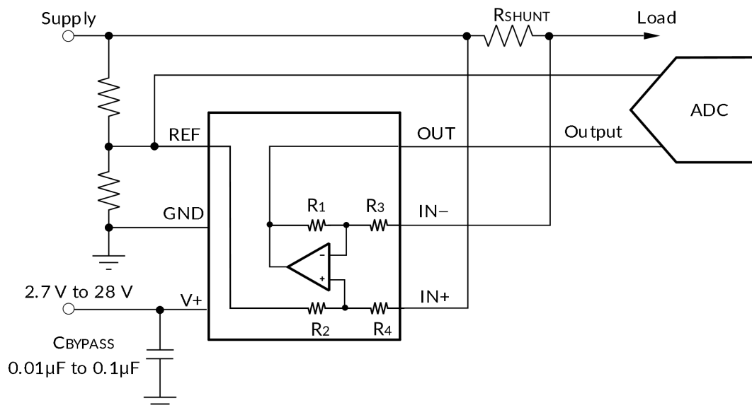
图 20. TLX199XP 消除阻抗对REF输入的影响
