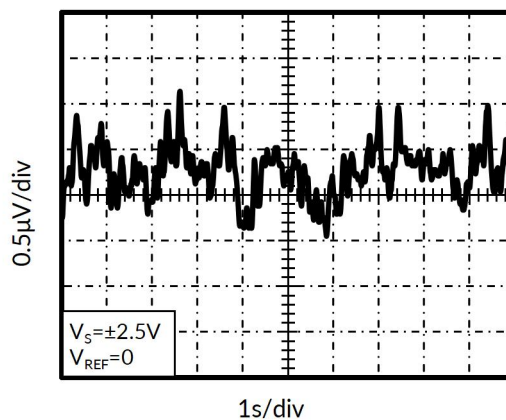
图 10. 0.1\text{Hz} \sim 10\text{Hz} 输入电压噪声
