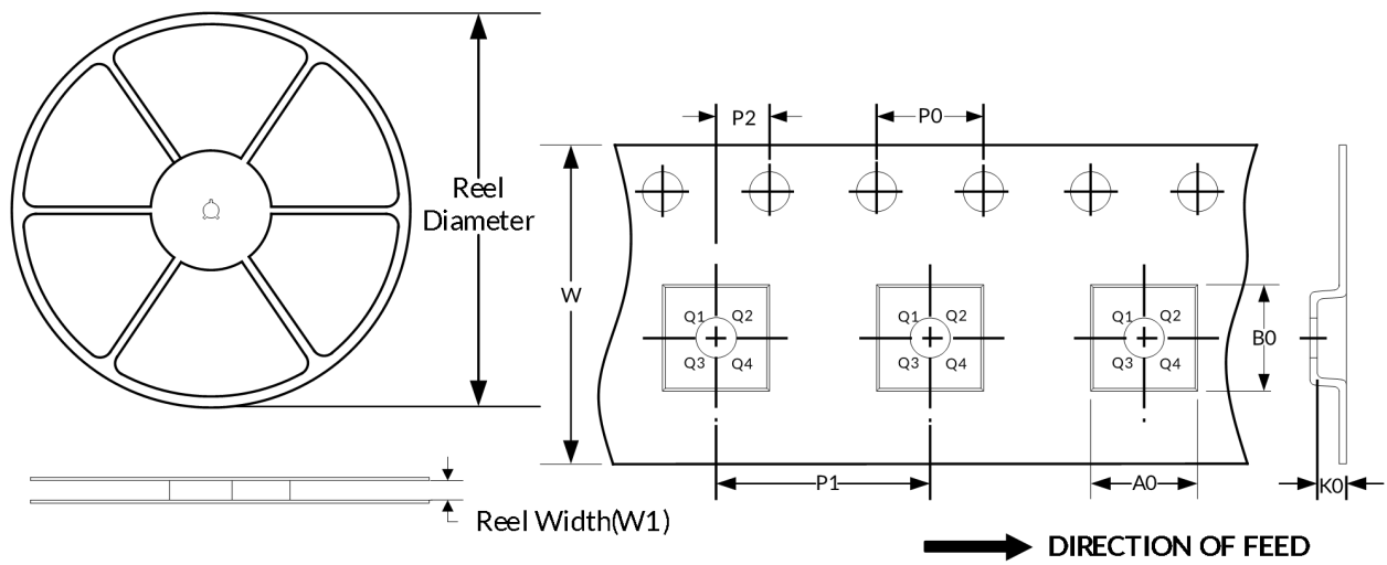
卷轴尺寸
