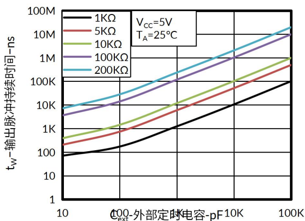
图 7. 输出脉冲持续时间与外部定时电容的关系
