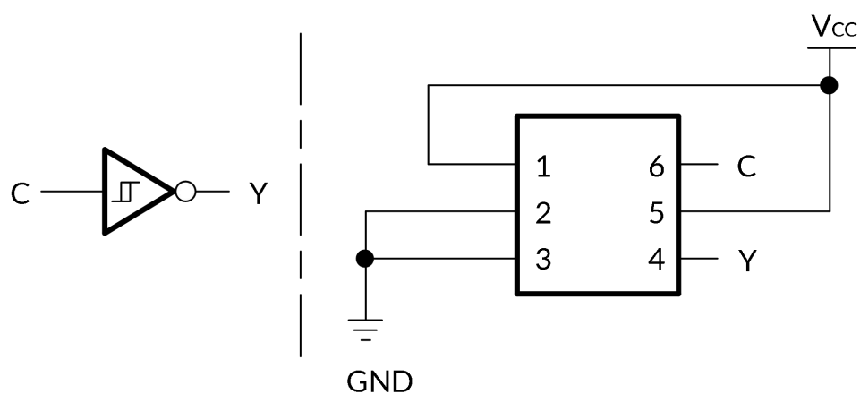
图 7. 反相器
