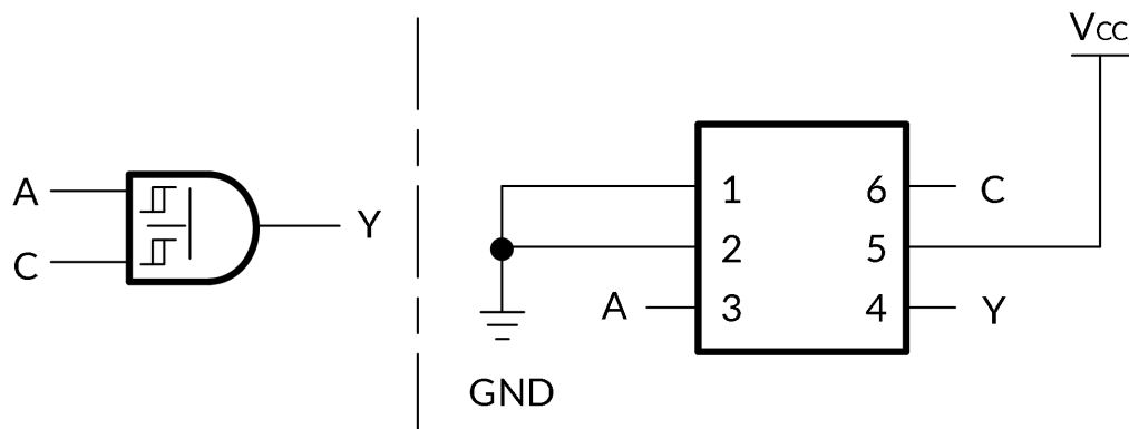
图 3. 两输入与门
