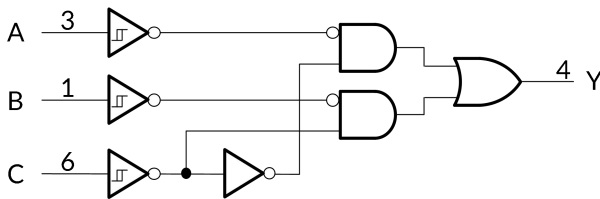
逻辑图示 (正逻辑)
