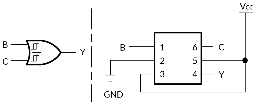
图 6. 两输入或门
