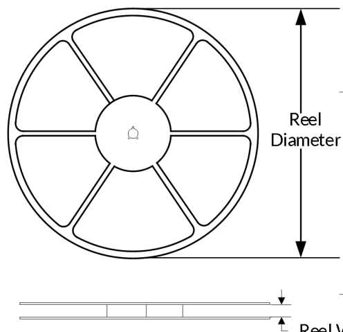
卷盘尺寸
