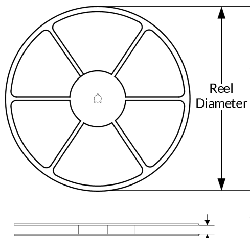
卷盘尺寸
