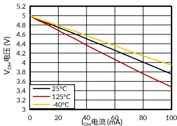
图 2. 电压与电流的关系
