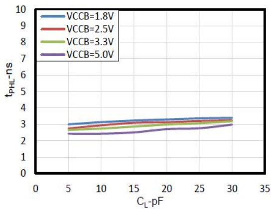
图 6. 高到低 (A 到 B) 典型传播延迟与负载电容的关系
