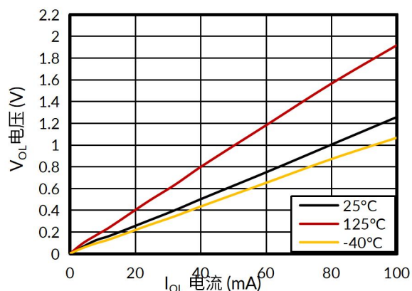
图 1. 电压与电流的关系
