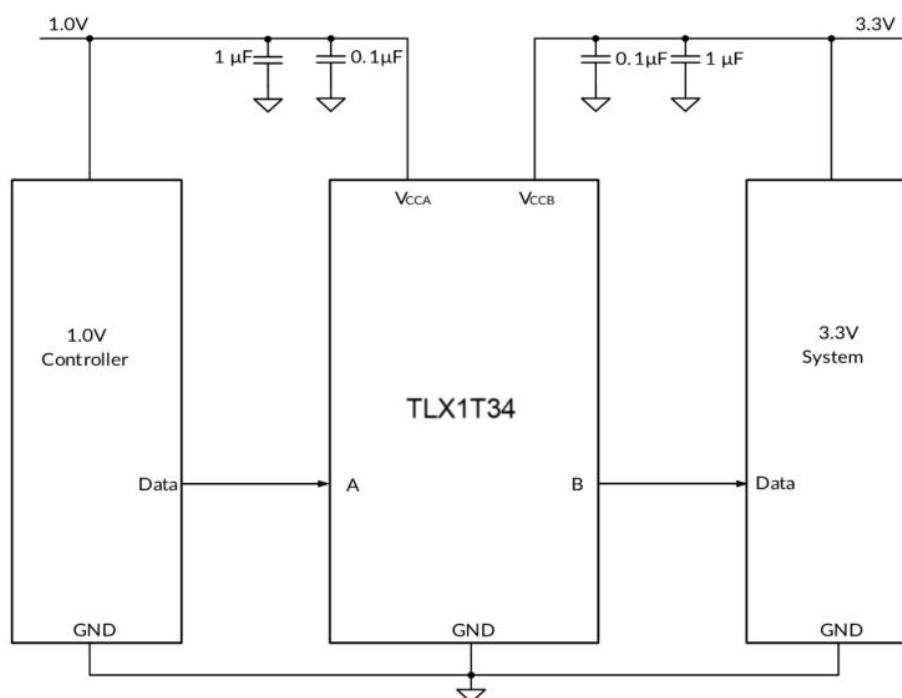
图 8. 典型应用电路
