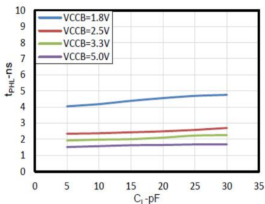
图 5. 高到低 (A 到 B) 典型传播延迟与负载电容的关系
