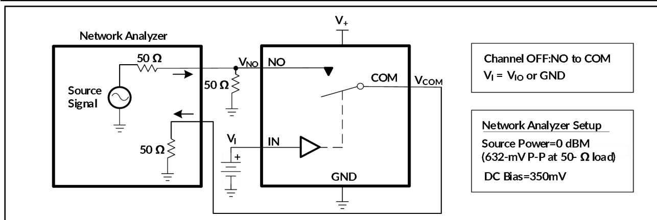
图 17. 关断隔离 ( O_{Iso} )
