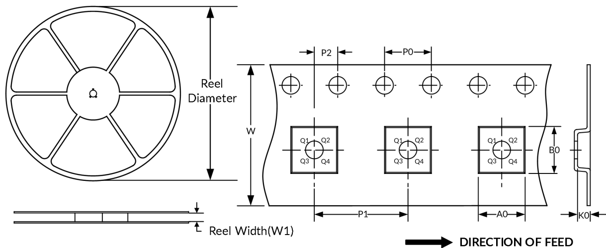
卷盘尺寸
