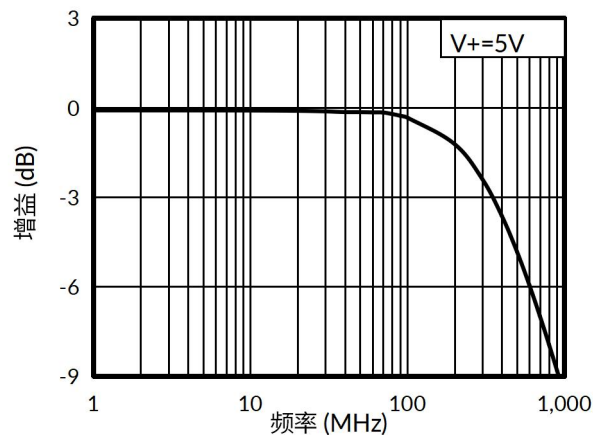
图 2. 带宽
