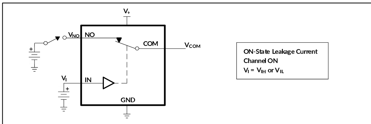
图 10. 导通漏电流 ( I_{COM(ON)} , I_{NO(ON)} )
