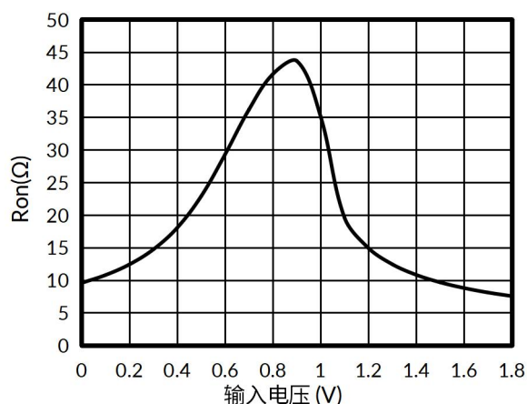
图 3. 导通电阻的典型值和输入电压的函数关系( V_+ = 1.8V )
