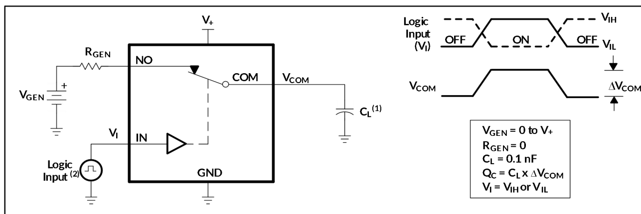
图 19. 电荷注入 ( Q_c )
