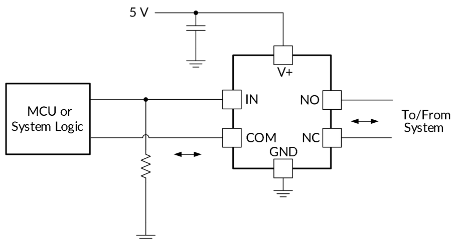
图 20. TLX2057A 系统原理图
