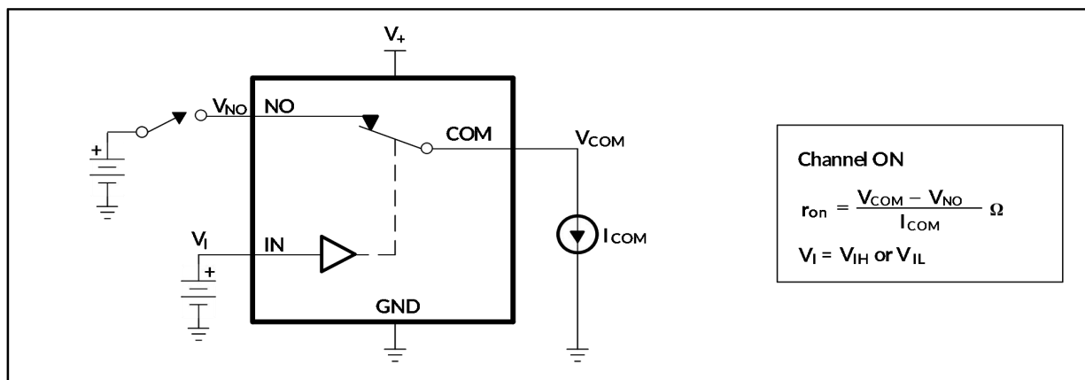
图 8. 导通电阻 ( R_{on} )
