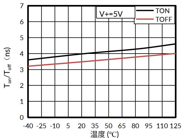
图 5. T_{on} 和 T_{off} 时间和温度的关系
