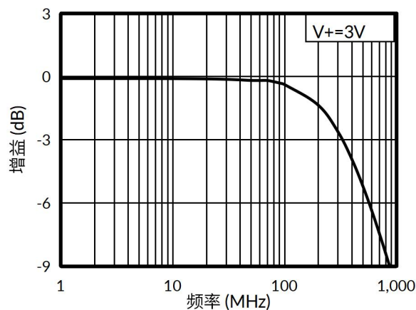
图 1. 带宽
