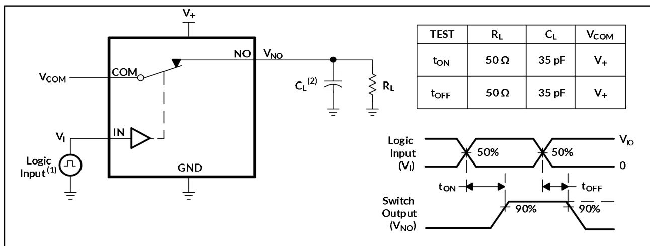
图 8. 启动 ( t_{ON} )和关断时间 ( t_{OFF} )
