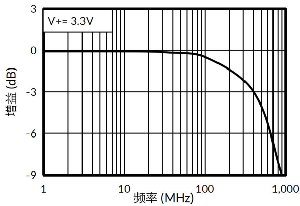
图 1. 带宽
