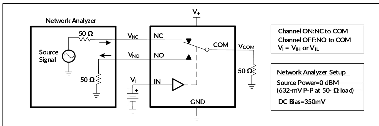
图 12. 串扰 ( X_{TALK} )
