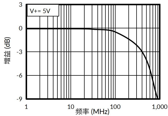
图 2. 带宽
