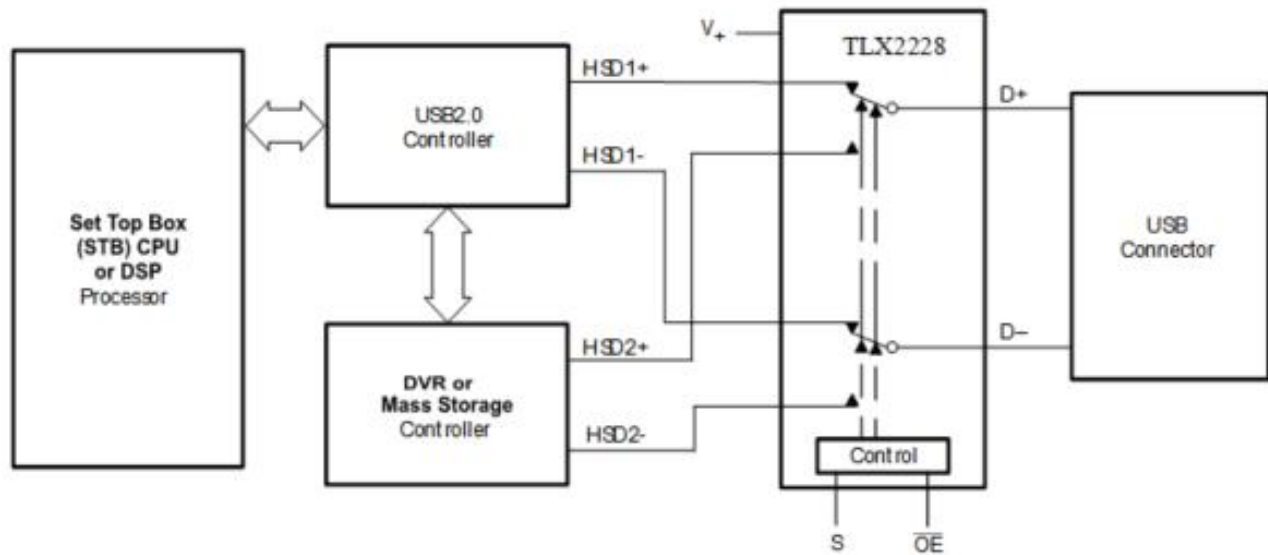
图 8. 应用框图
