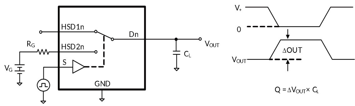
图 7. 电荷注入量 (Q)
