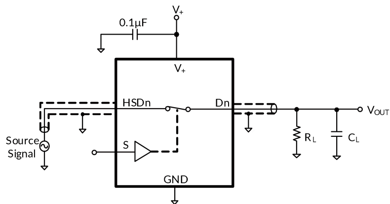
图 6. -3dB 带宽
