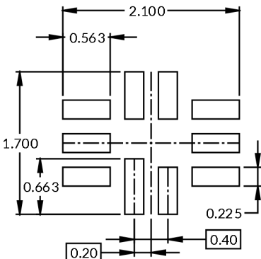
推荐焊盘尺寸
