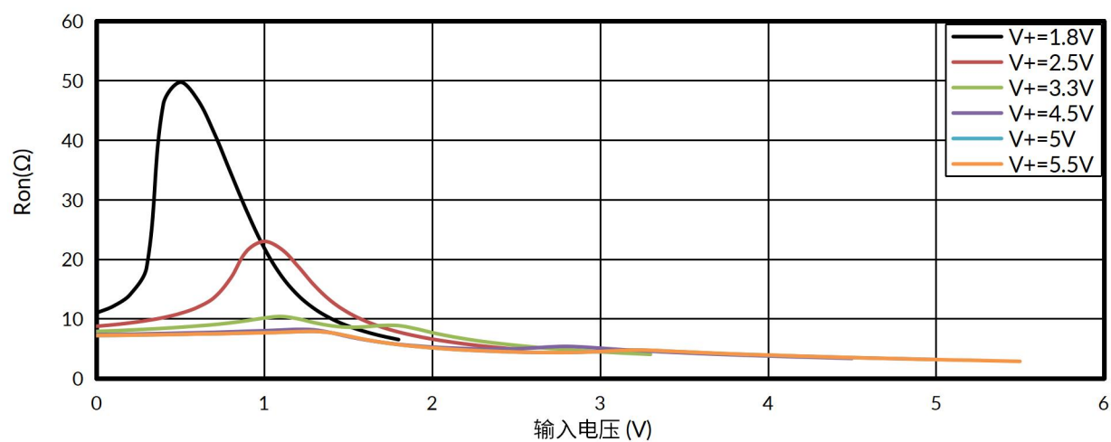
图 1. 导通电阻 ( R_{on} ) 的典型值和输入电压的函数关系
