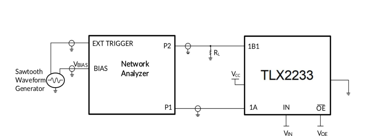
测试电路 1. 电压波形和开关时间测试电路
