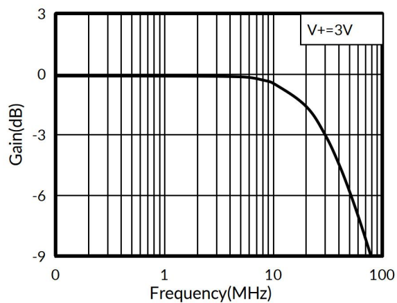
图 1. 带宽与频率
