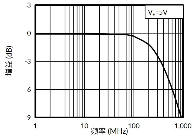
图 2. 带宽
