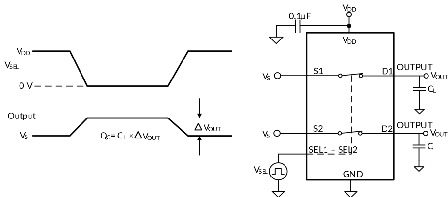
图 11. 电荷注入 (Qc)
