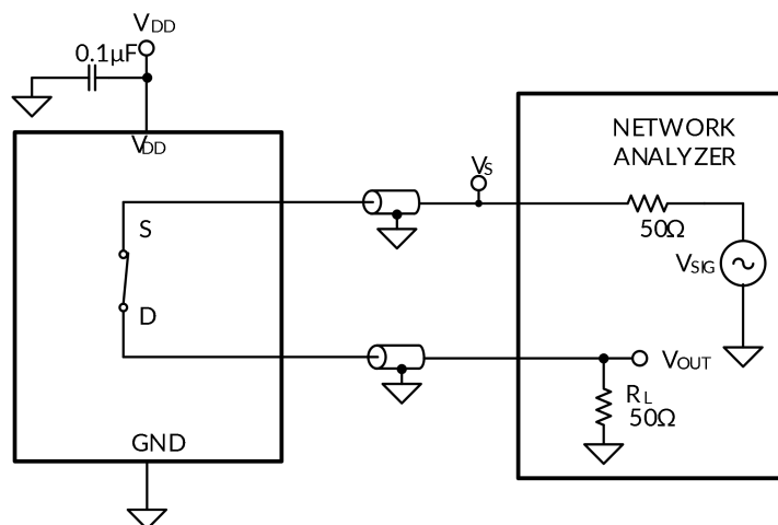
图 8. 带宽 (BW)
