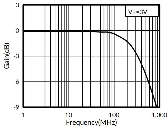
图 1. 带宽与频率
