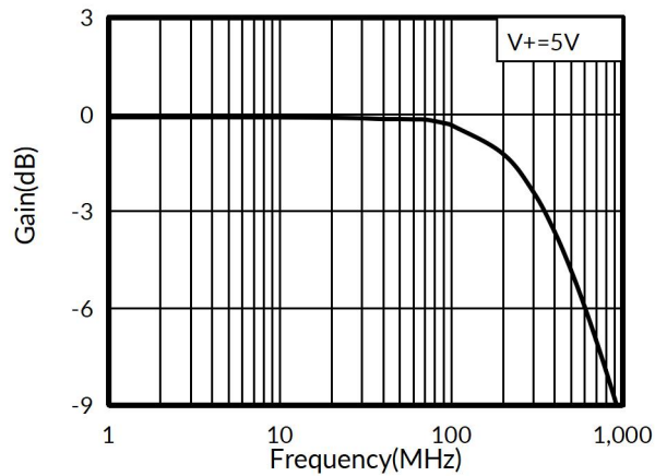
图 2. 带宽与频率
