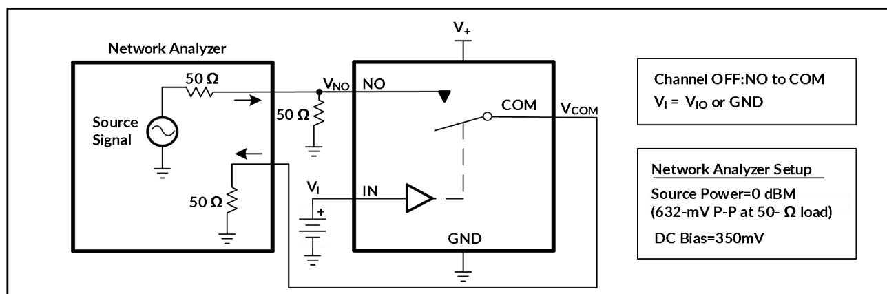
图 11. OFF 隔离 (O ISO )
