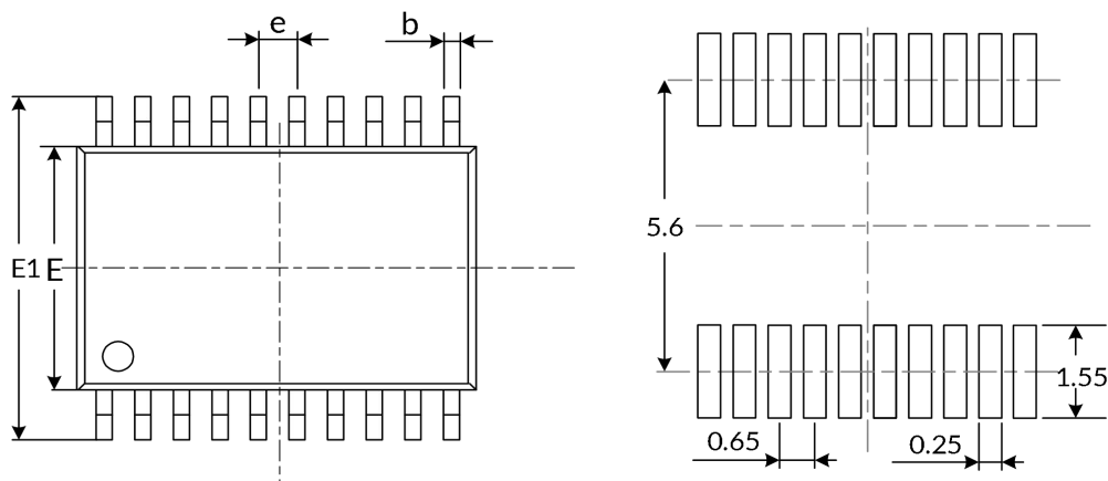
推荐焊盘尺寸 (单位: 毫米)
